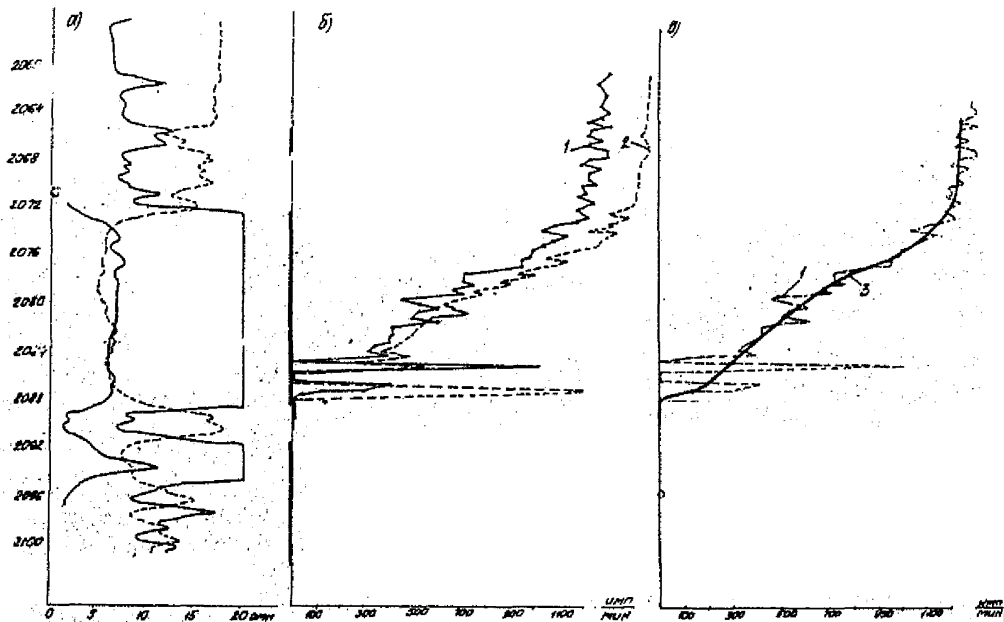
Рис. 26. Пример коррекции профиля. а) каротажные диаграммы, б) некорректированные профили на двух режимах-1 и 2, в) скорректированный профиль - 3
