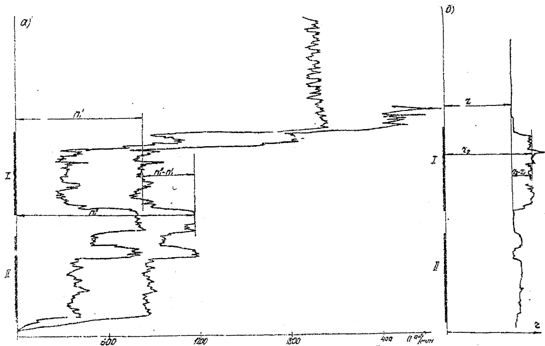
Рис. 27. I-2- перфорируемые пласти; n' , n'' -числа оборотов турбинки при одинаковых расходах в перфорируемой и n же перфорируемой зонах; z_1, z_2 -радиусы колонны.
