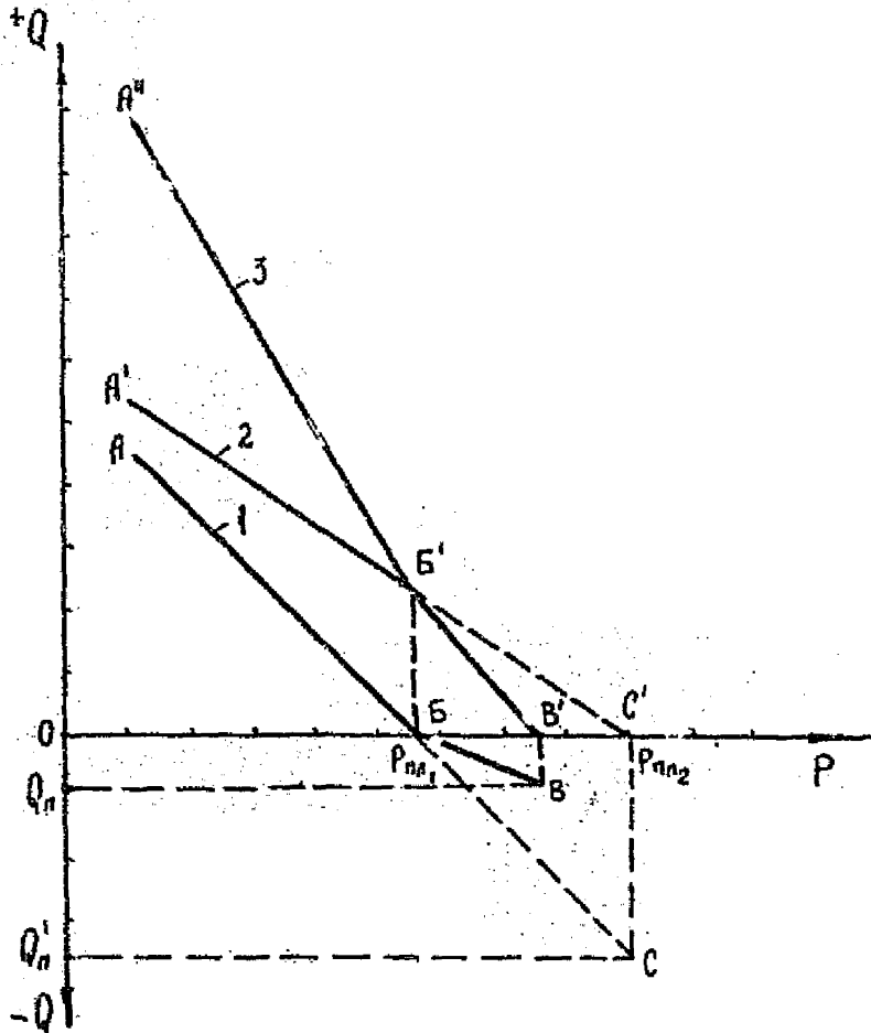
Рис. 33. Индикаторные кривые
