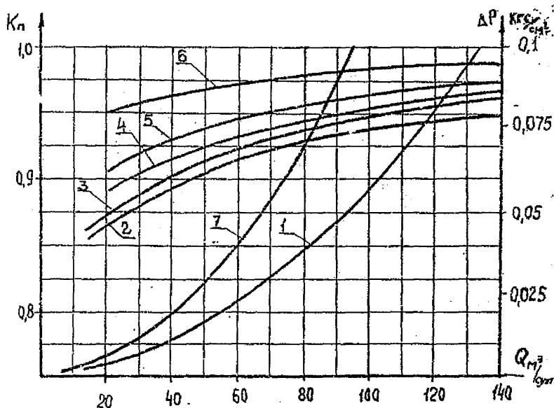
Рис. 8. Зависимость коэффициента поправки "ПОТОК-5" и перепада давления на приборе от расхода жидкости различной вязкости.
