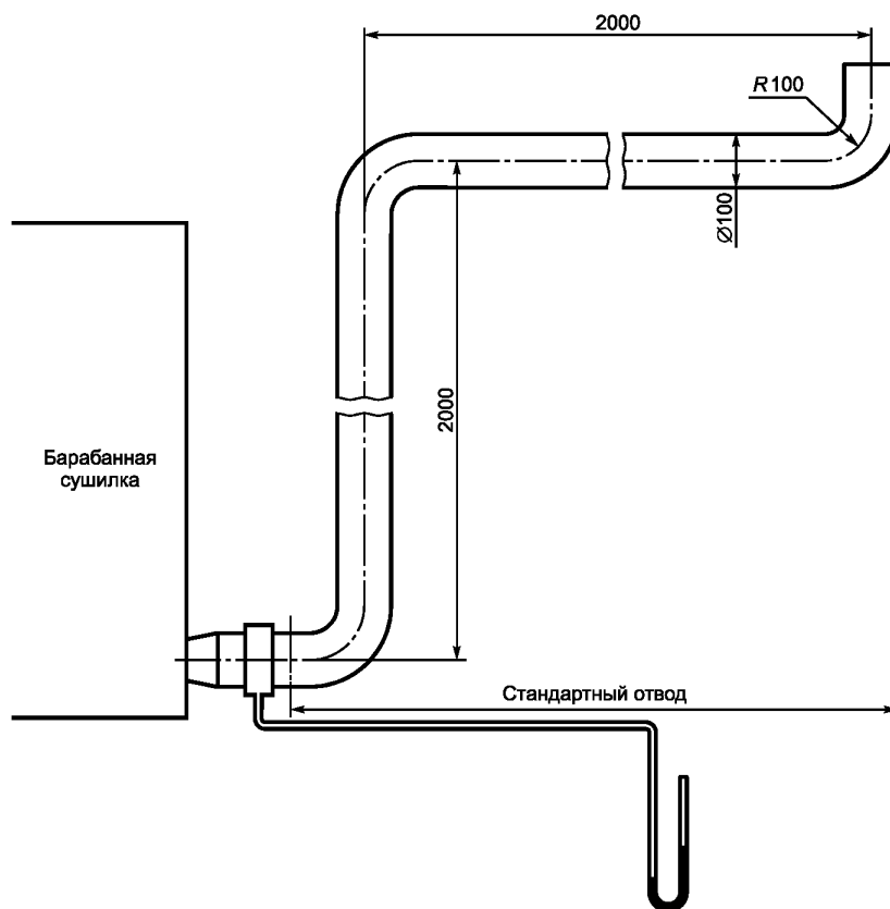
Рисунок А.2 — Стандартный отвод
