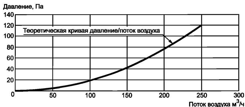
Рисунок А.1 — Кривая давление/поток воздуха
