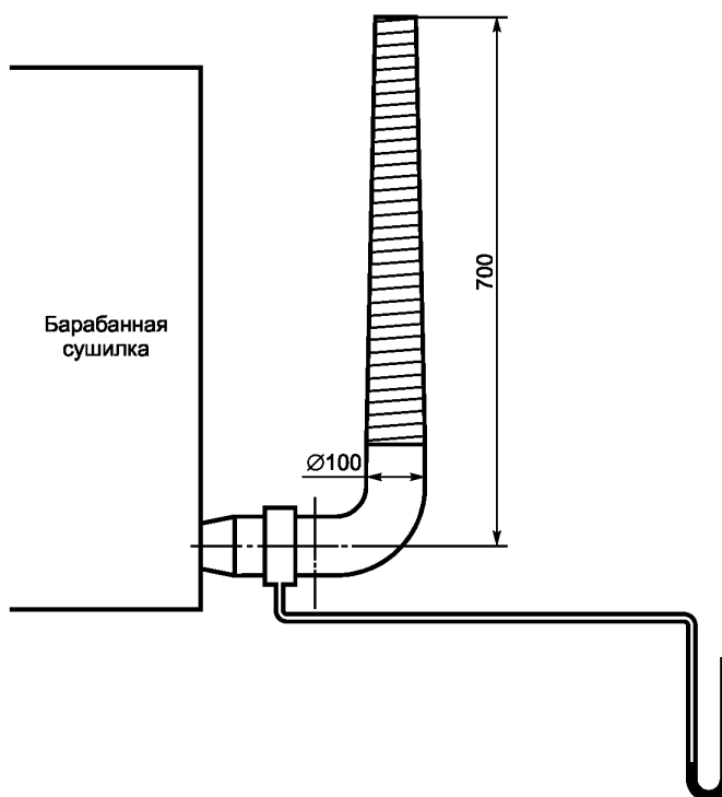
Рисунок А.3 — Имитатор стандартного отвода
