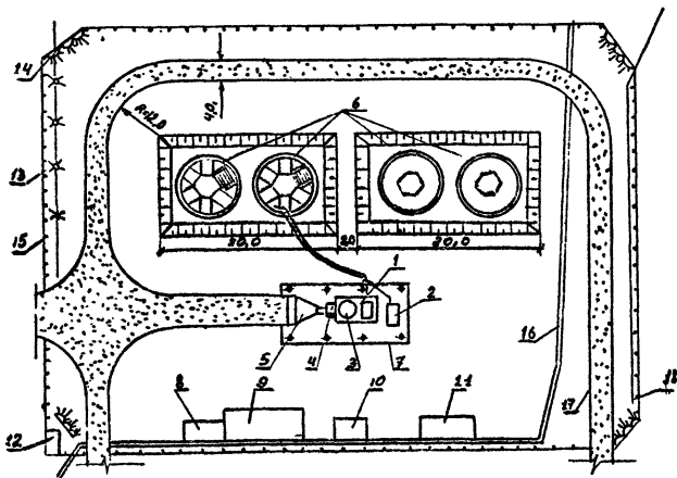
Рис.1. Стрейфенплан (на период пневмобетонирования стян резервуара);
