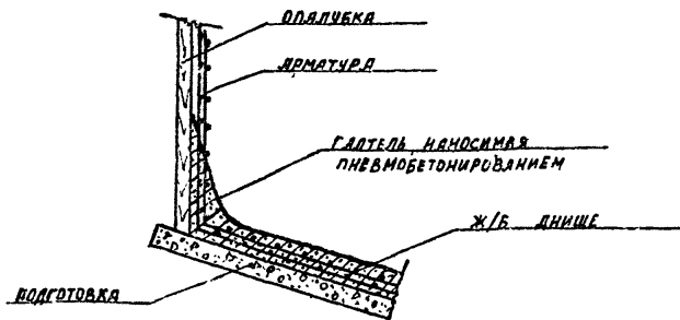
Рис.3. Устройство галтели.
