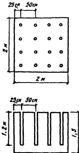
Рис.4. План расположения шпуров при разрушении бетонного фундамента
