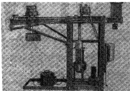
Рис.2. Установка для измерения давления расширения
