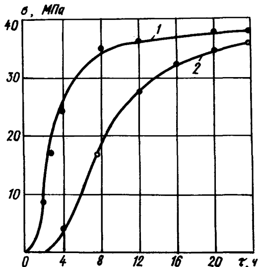
Рис.3. Кинетика развития давления расширения при твердении образцов НРВ кривая 1 - состав I; кривая 2 - состав 2
