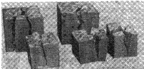
Рис.1. Характер разрушения бетонных образцов с помощью НРВ
