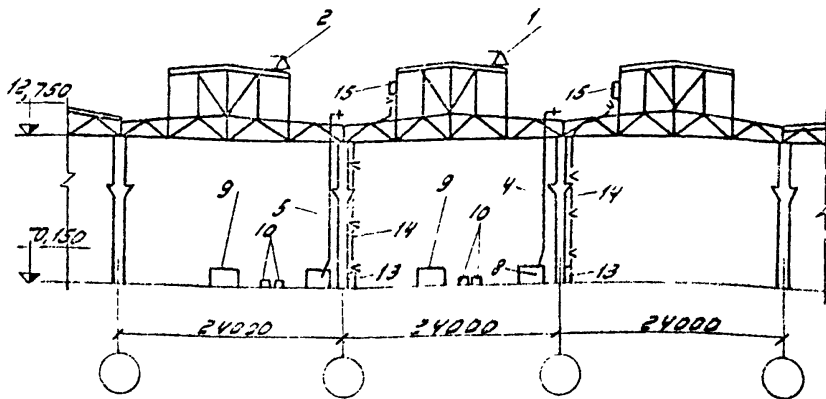
Рис. 2. Разрез А-А
