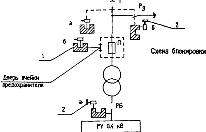
Оперативная схема блокировки
