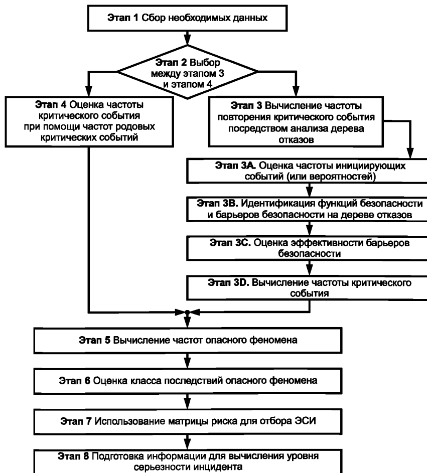
Рисунок 1 — Общая схема этапов МИЭСИ
