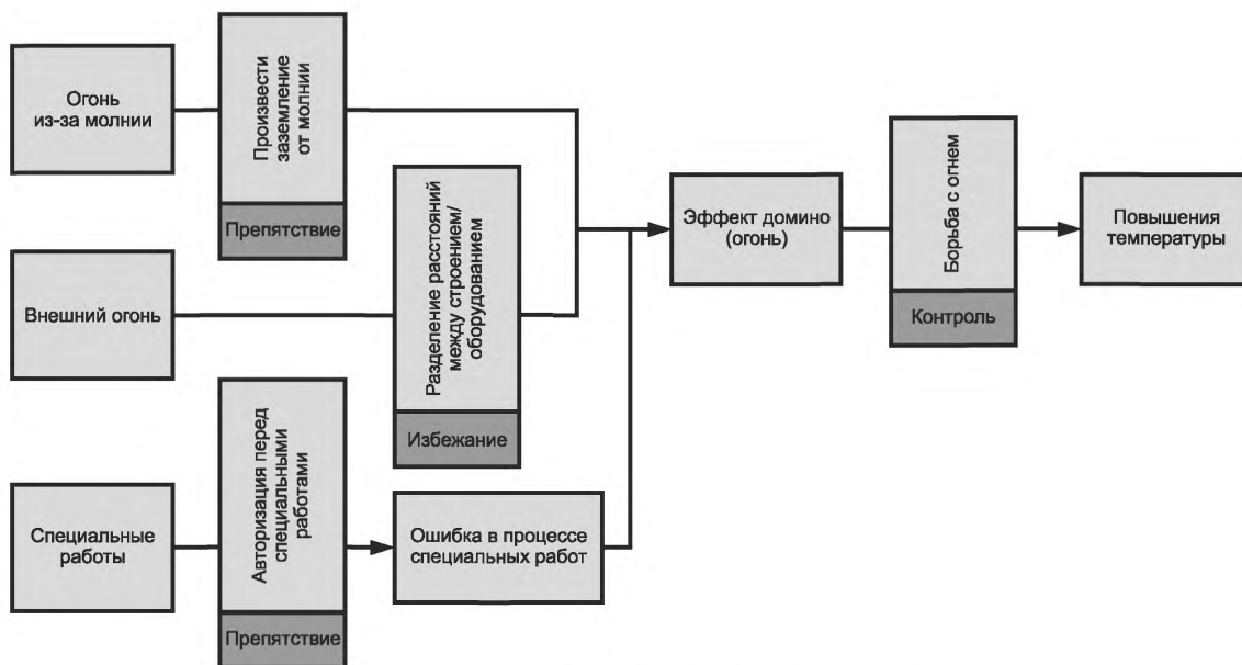
Рисунок 2 — Барьеры, размещенные на ветвях дерева отказов
