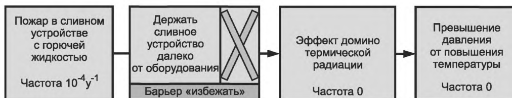
Рисунок 3 — Барьер «избежать»
