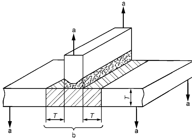
a — стрелки указывают направление нагрузки; b — заштрихованная область показывает охват ультразвукового контроля
