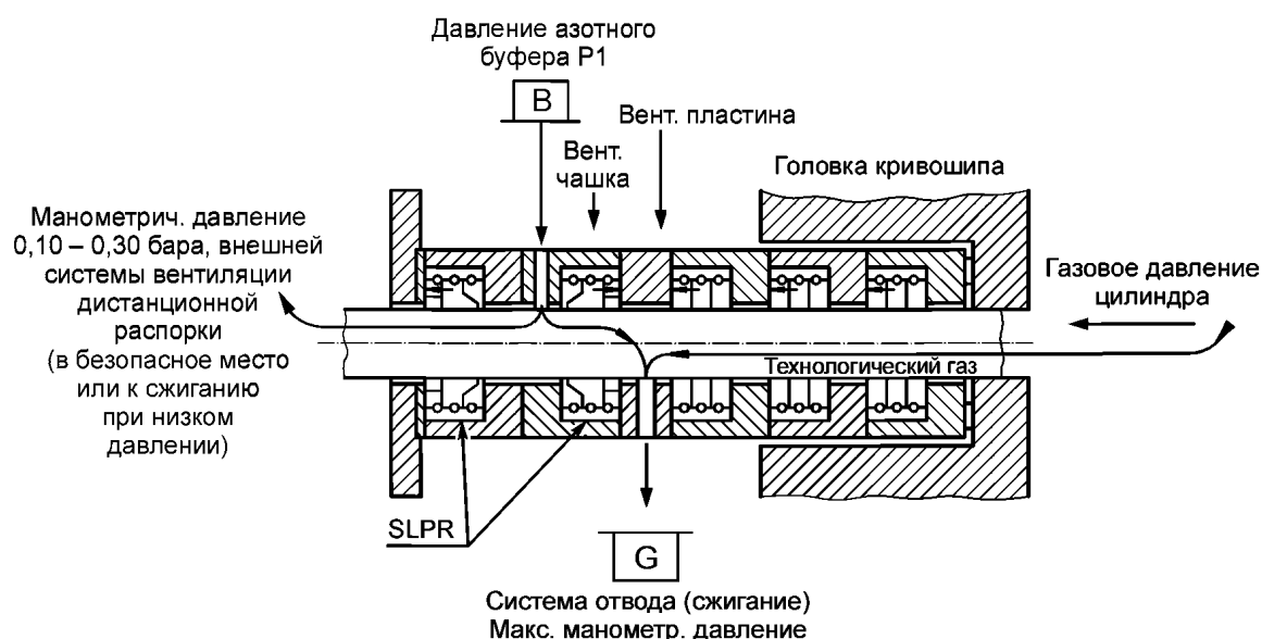
Прижимное уплотнение
