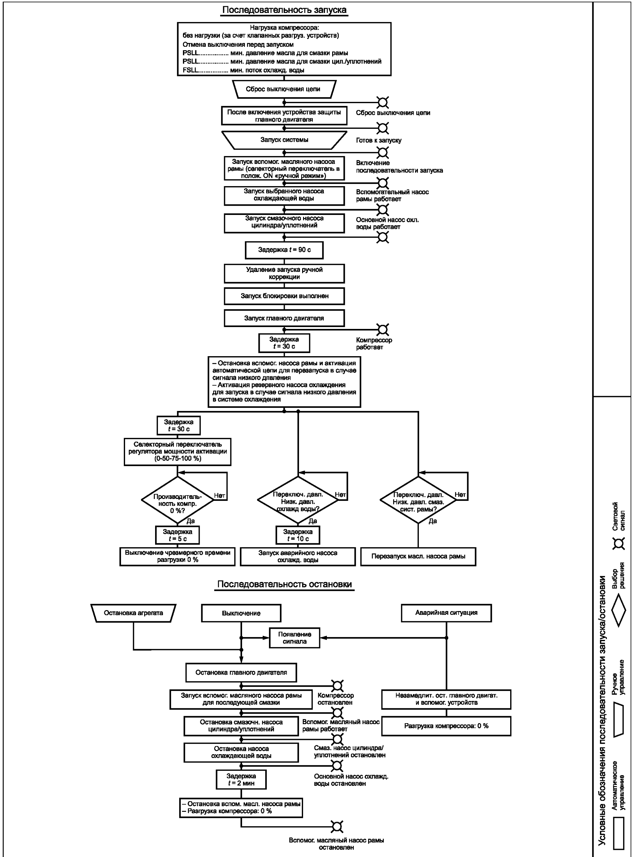
Рисунок Е.6 — Типовая логическая схема автоматического пуска/останова
