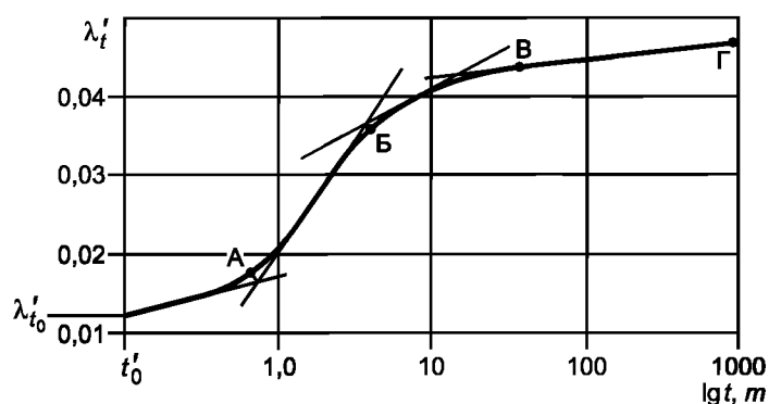
Рисунок К.2 — Определение границ этапов консолидации
