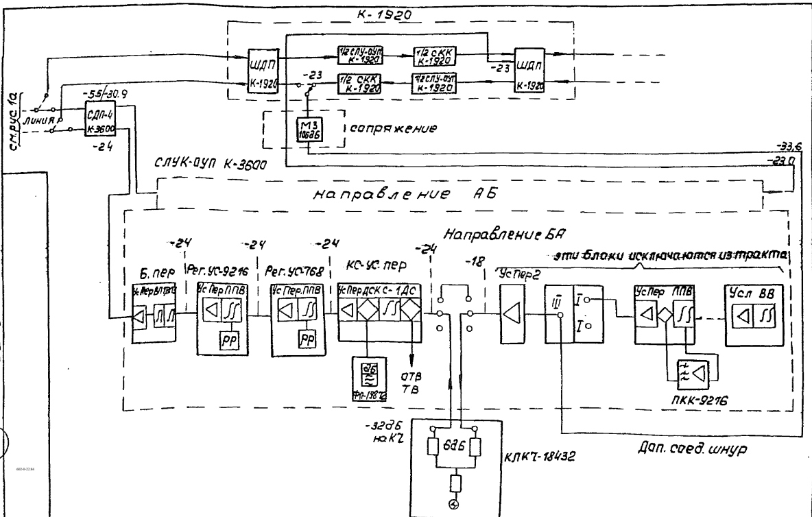
Рис 16 Схема сопряжения линейных трактов К-1920 с К-3600 в ОУП
