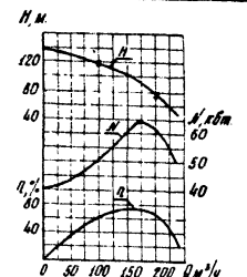
Характеристика насоса 34Б 12-160-100
