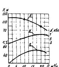
Характеристика насоса 3ЦДБ 8-16-110
