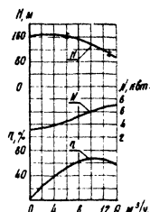
Характеристика насоса 13ЦДБ 6-10-140
