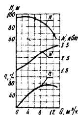
Характеристика насосов 3ЦДБ 6-10-60 и 13ЦДБ 6-10-60
