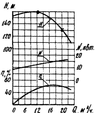
Характеристика насосов 3ЦДБ 8-25-150 и 3ЦДБ 8-25-150Г
