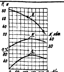
Характеристика насоса 34Б 12-210-55
