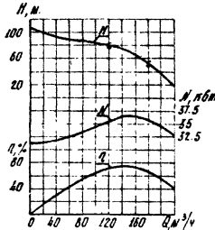
Характеристика насоса 34Б 10-160-65
