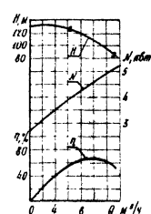
Характеристика насоса 3ЦДБ 6-10-110
