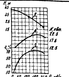
Характеристика насоса 34Б 12-210-25
