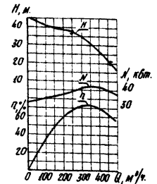
Характеристика насоса 34Б 12-315-30
