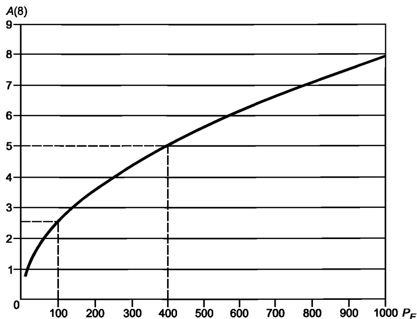
Рисунок 1 — Соотношение между индексом вибрационной экспозиции P_E и вибрационной экспозицией за смену A(8)
