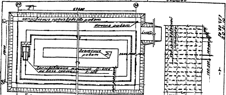
Схема уплотнения грунта трамбовочной машиной П-471Б
