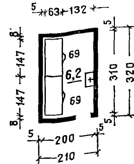
Гардеробная персонала для баз отдыха вместимостью 500 мест
