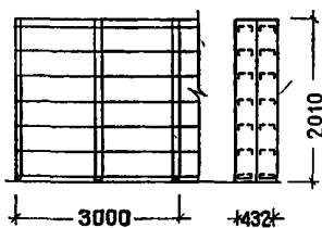
24 Стеллаж книжный двухсторонний
