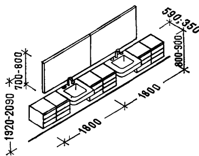
⑥ Туалет парикмахерский с умывальником
