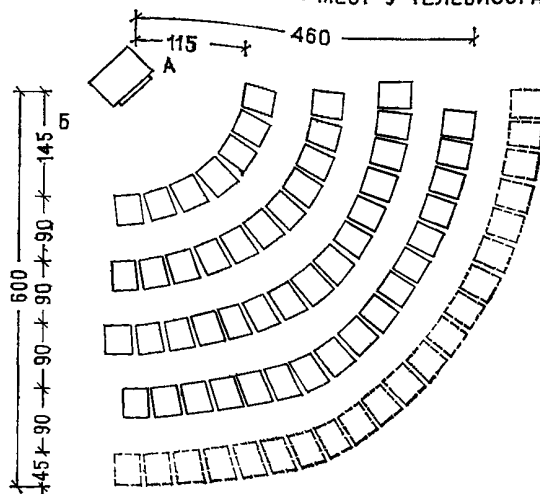
ГРУППИРОВКА ЗРИТЕЛЬСКИХ МЕСТ У ТЕЛЕВИЗОРА
