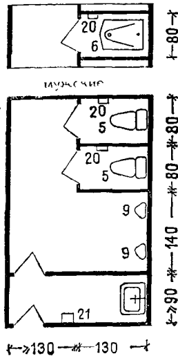
Общие санитарные узлы Уборные с умывальником в шлюзе на 50 человек
