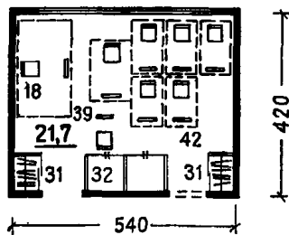
Музыкальный кружок Эстрадный оркестр на 8 человек
