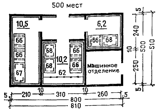
Кладовая овощей, квашений и солений для баз отдыха вместимостью 250 мест 500 мест
