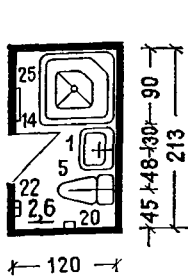
Общие санитарные узлы Уборные с умывальником в шлюзе на 50 человек
