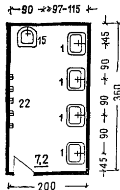
Умывальная с ножной ванной на 50 женщин или 100 мужчин
