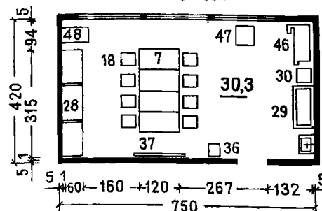
Универсальное использование помещения для артистов под кружковые помещения Помещения для артистов
