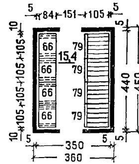
Кладовая сухих продуктов для баз отдыха вместимостью 250 мест 500 мест
