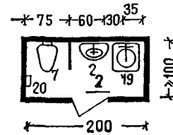
Туалетная для детей на 50 мест
