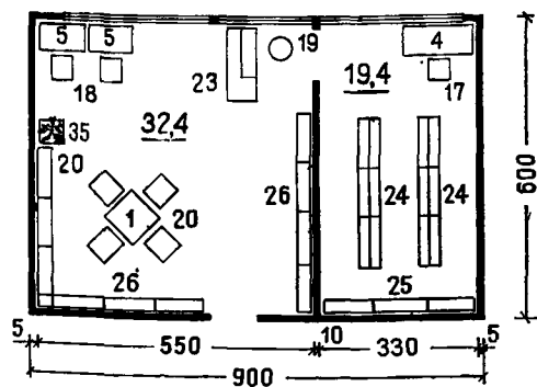
БИБЛИОТЕКА НА 10000 КНИГ ДЛЯ БАЗ ОТДЫХА ВМЕСТИМОСТЬЮ 1000 мест
