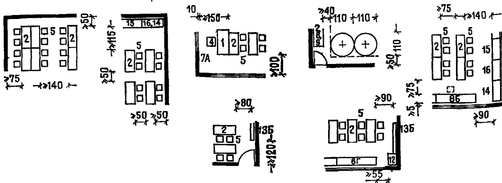
Индивидуальные занятия, игры
