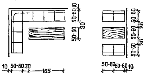
Пристенное расположение мебели
