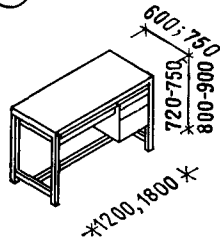
⑨ Стол приемщика
