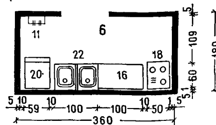
Буфетная на 500 отдыхающих
