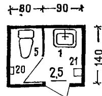
Умывальная с ножной ванной на 50 женщин или 100 мужчин
