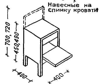
⑥ Подставка для чемо- данов складная
