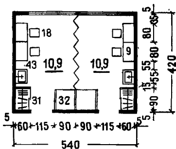
Изокружок на 8 человек
