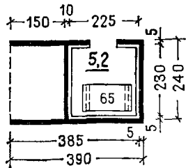
Камера отходов для баз отдыха вместимостью 250 и 500 мест
