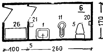
Кабина личной гигиены женщин
