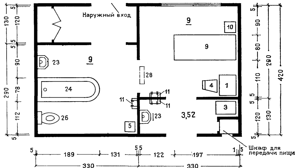
Палата на 1 койку
