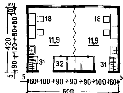
Универсальное использование помещения для артистов под кружковые помещения Помещения для артистов
