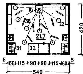
Музыкальный кружок Эстрадный оркестр на 8 человек
