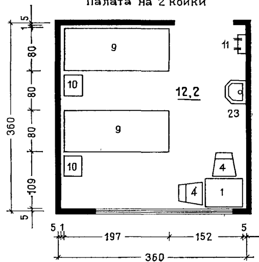
Палата на 2 койки
