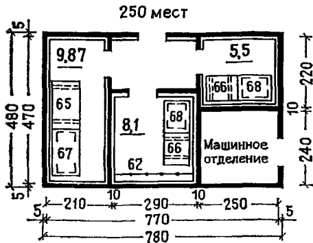
Камера отходов для баз отдыха вместимостью 250 и 500 мест
