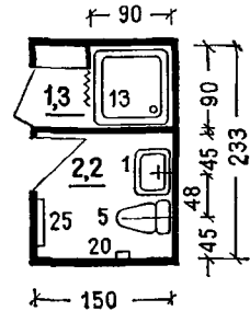
Туалетная для детей на 50 мест
