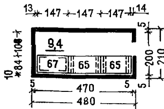
Кладовая инвентаря для баз отдыха вместимостью 250 и 500 мест
