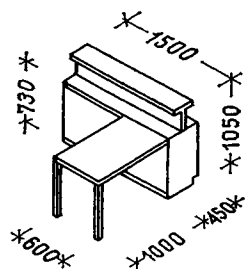
①,2 Барьер регистратора со столом-приставкой
