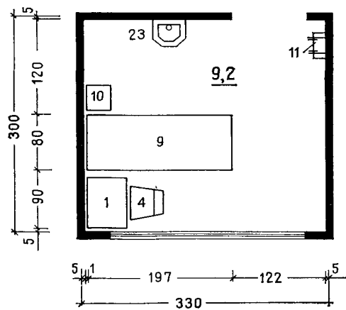
Палата на 1 койку
