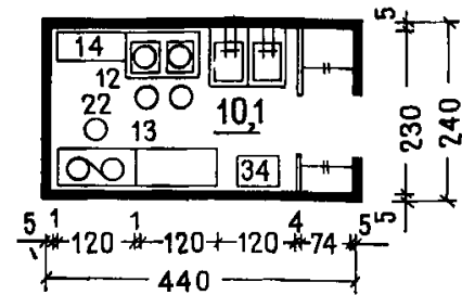
Кинофотолаборатории для баз отдыха вместимостью 500 и 1000 мест
