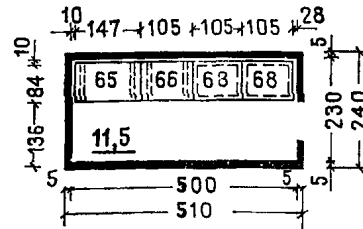
Кладовая суточного запаса для баз отдыха вместимостью 500 мест
