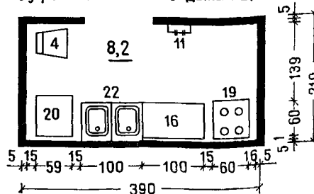
Буфетная на 1000 отдыхающих
