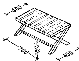
⑥ Подставка для чемо- данов складная
