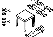
⑮ Стол журнальный блокируемый
