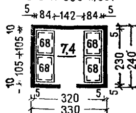
Кладовая инвентаря для баз отдыха вместимостью 250 и 500 мест
