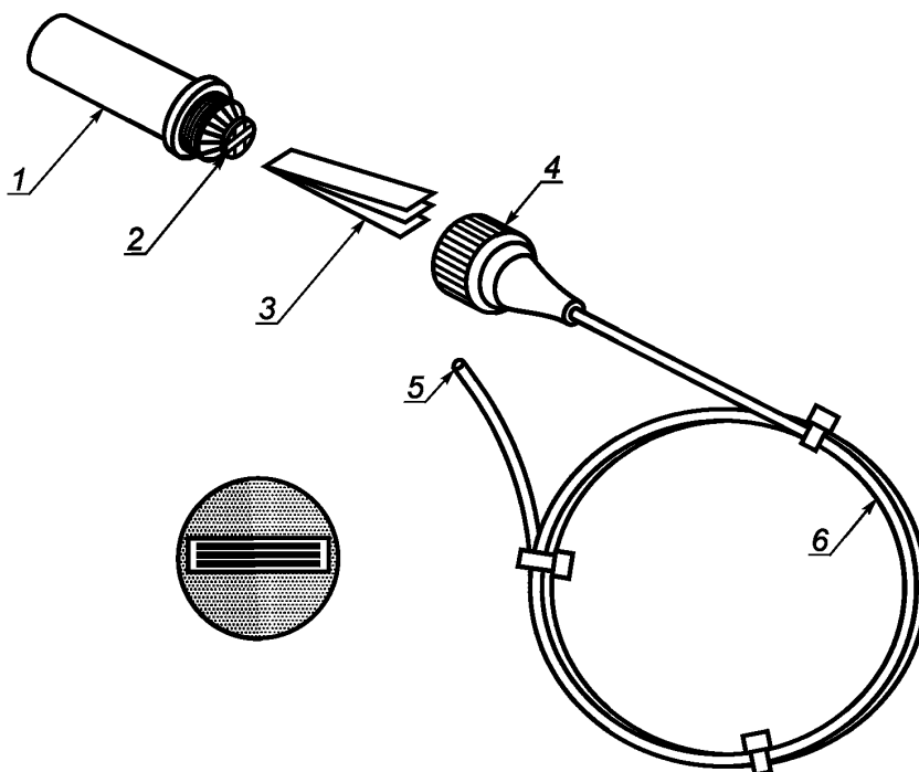
1 — капсула; 2 — уплотнение; 3 — индикаторная система; 4 — разъем; 5 — открытый конец; 6 — трубка
