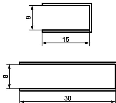
Рисунок А.2 — Полые объекты типа А
