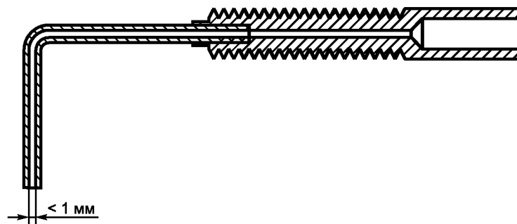
Рисунок 10 — Проходной фитинг
