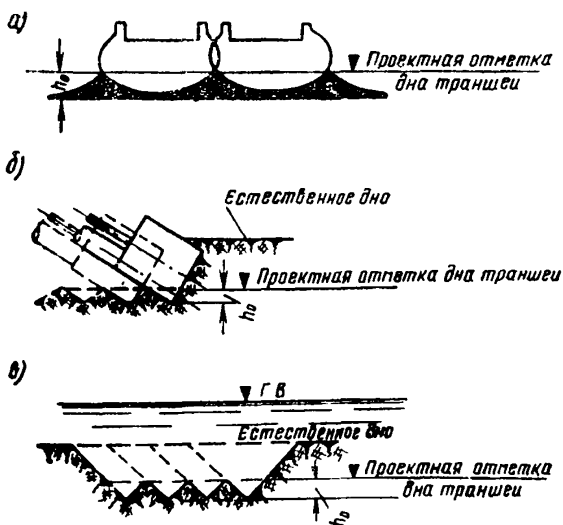
Рис. 1. Схемы разработки траншей земснарядами: а—многочерпаковым; б—папилонажным; в—траншейным Примечание. h_n —допускаемый перебор грунта
