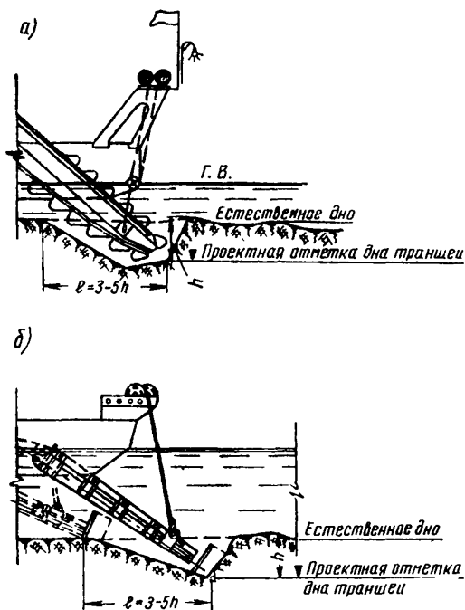
Рис. 2. Схема врезки в траншею земснаряда: а—многочерпакового; б—папильонажного Примечание. h —толщина срезаемого слоя грунта
