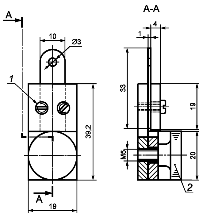
а) зажим
