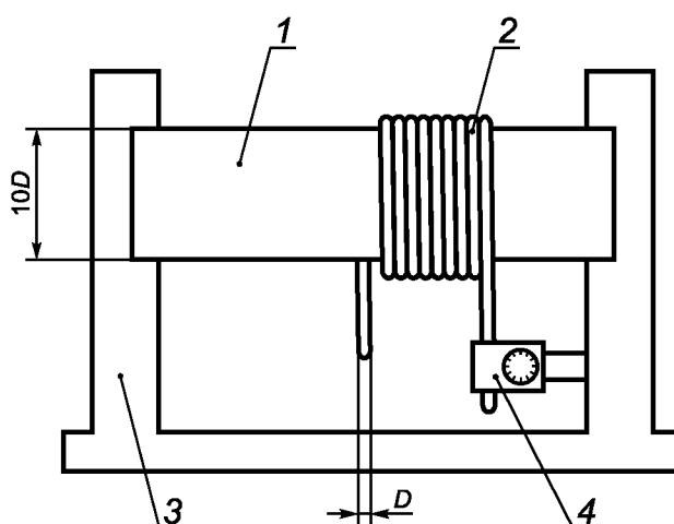
1 — цилиндрический валик; 2 — проводник; 3 — опоры; 4 — зажим
