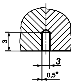
б) место крепления проводника (увеличено)
