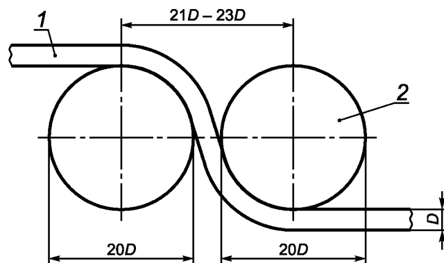
1 — проволочный проводник; 2 — цилиндрический валик
