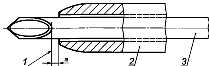
1 — кромка скоса иглы; 2 — интродьюсерный катетер; 3 — интродьюсерная игла
