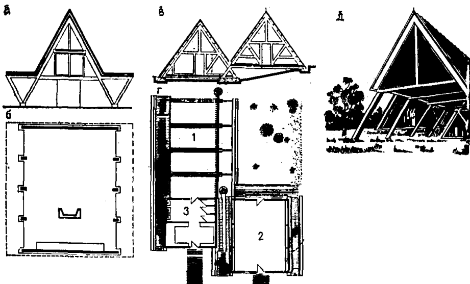
Рис 20. Игровые навесы и павильоны
