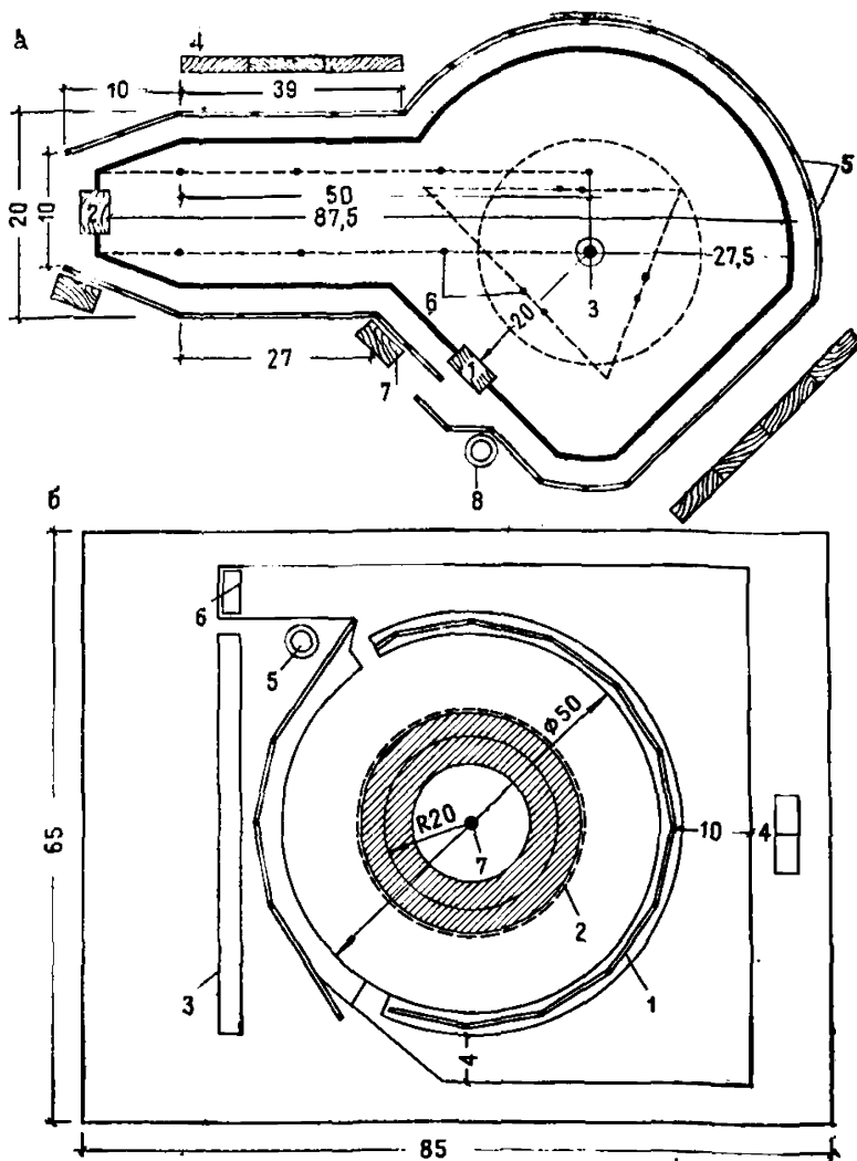
Рис. 31. Площадки для испытания моделей
