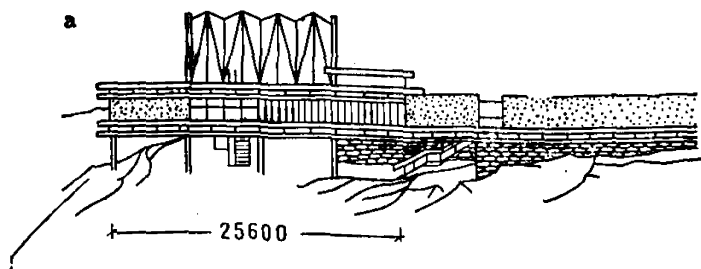
Рис. 23. Дом детского творчества пионерского лагеря на 400 мест в Алуште (КиевЗНИИЭП)
