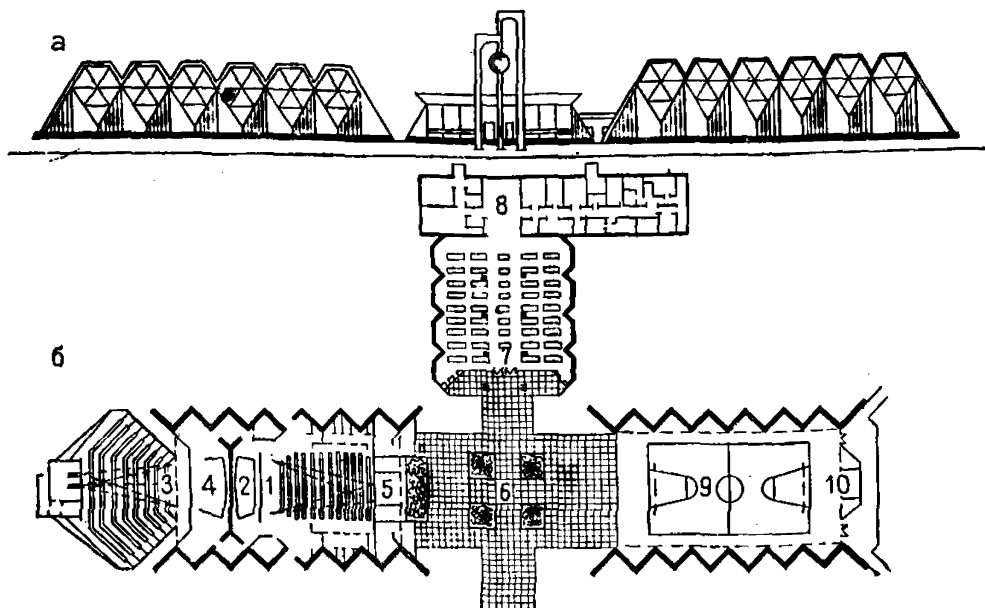
Рис. 24. Общественный центр. Экспериментальный проект ОЛС на 400 мест № 1-147 (ЦНИИЭП КТК)
