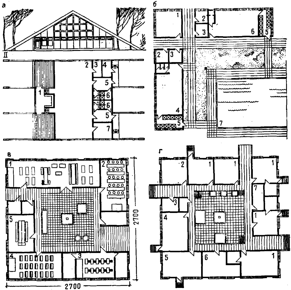
Рис. 30. Блоки помещений для специализированных занятий в ОЛС
