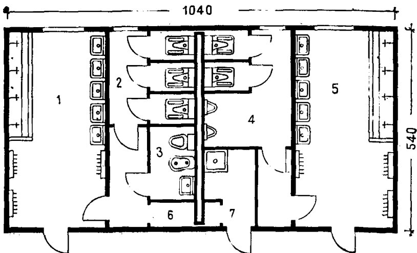
Рис. 7. План санитарно-технического павильона на два отряда
