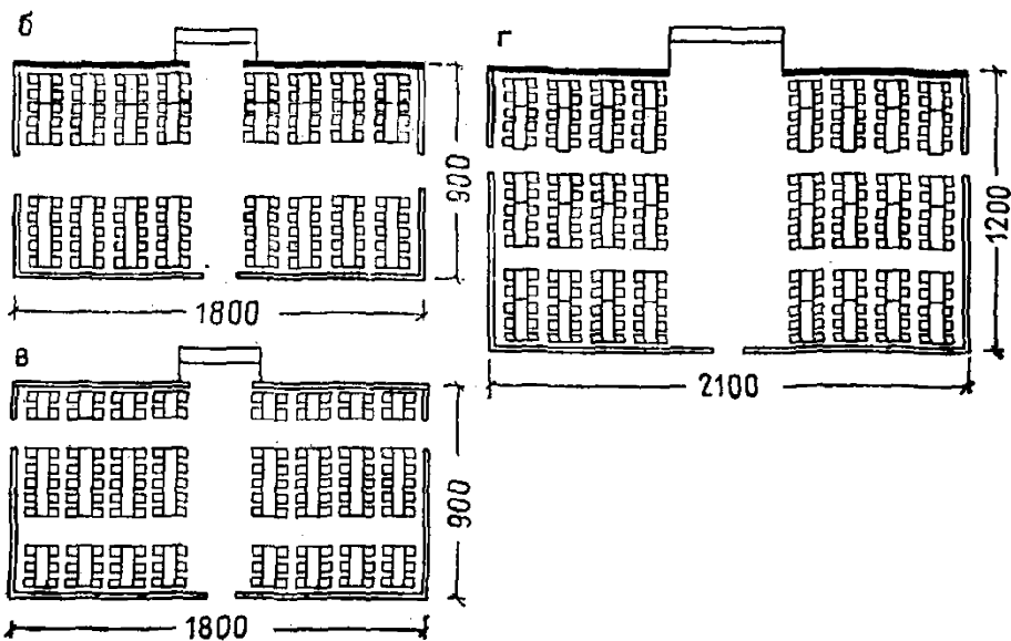
Рис. 18. Схемы размещения оборудования в обеденных залах ОЛС
