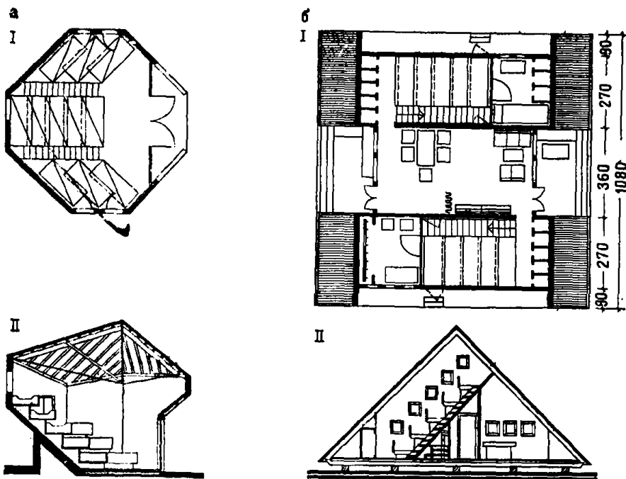
Рис 9. Летние домики со ступенчатым размещением спальных мест Домик загородного центра в Нара (Япония) (а) и домик на два звена по 5 чел. (предложение канд. архит. М. И. Магидиной) (б); I — план; II — разрез
