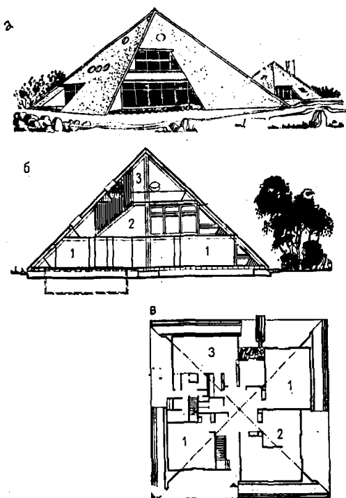
Рис. 38. Павильон общественного назначения детского центра отдыха в Ся-Филибер (Франция)
