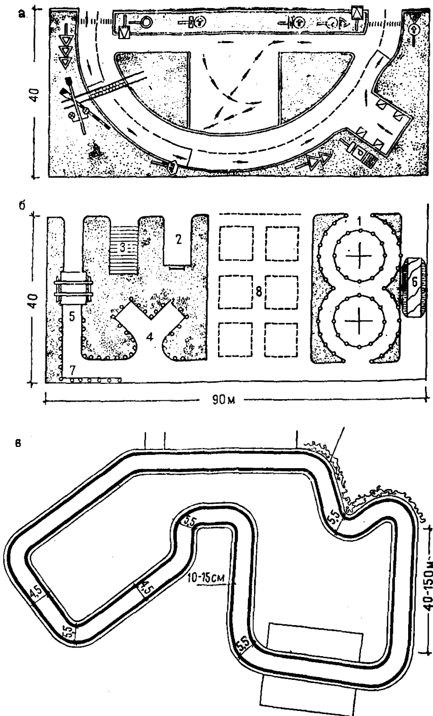
Рис. 28. Площадки для обучения вождению автотранспорта a — площадка для изучения правил дорожного движения; б — площадка для начального обучения практическому вождению автомобиля: 1 — восьмерка; 2 — щитовая погрузочная аппарель; 3 — торцевая возвышенная погрузочная аппарель с въездом; 4 — «ласточкин хвост»; 5 — железнодорожный переезд; 6 — разбитый участок маршрута; 7 — Г-образный проезд; 8 — площадка для изучения дорожных знаков; в — разметка трассы картинга
