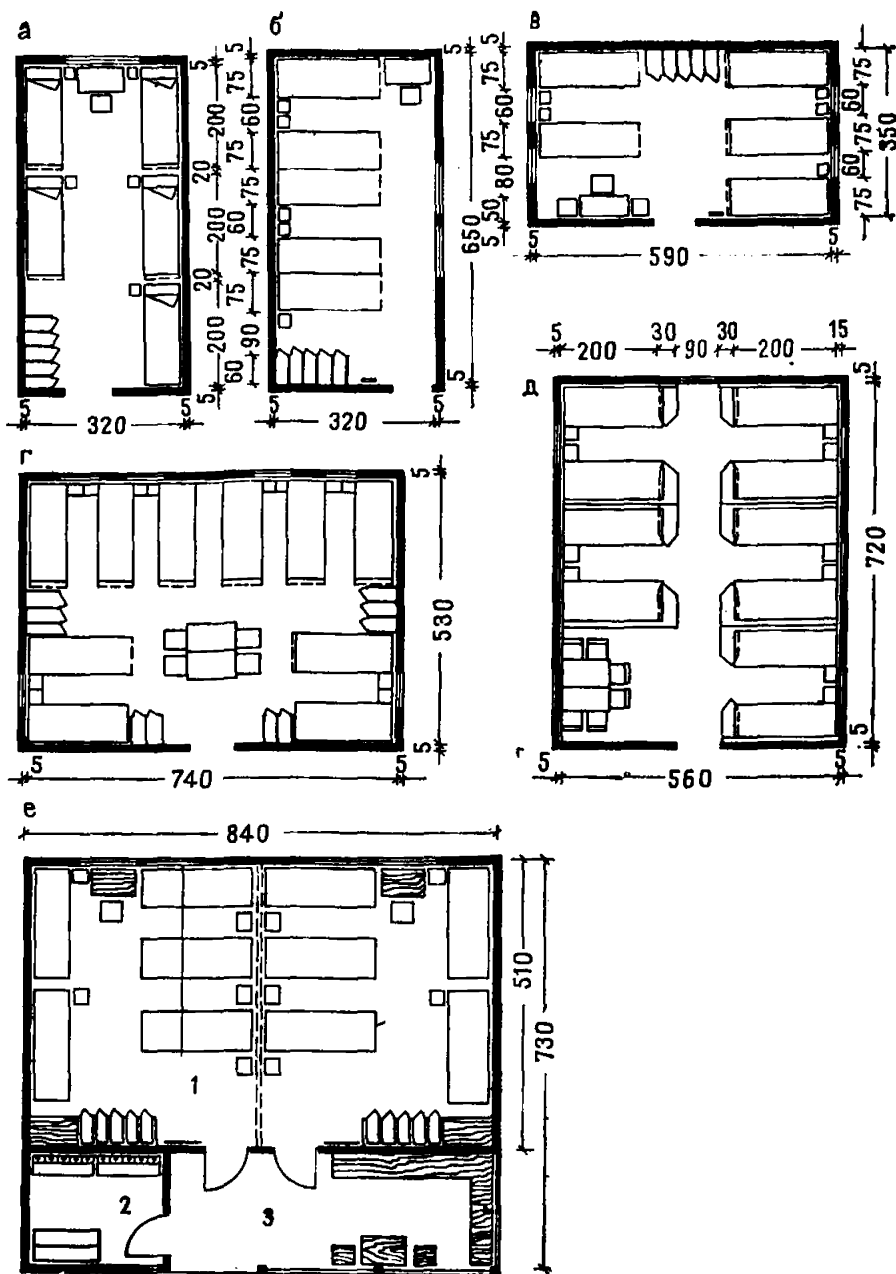
Рис. 5. Оптимальные габариты спальных комнат
