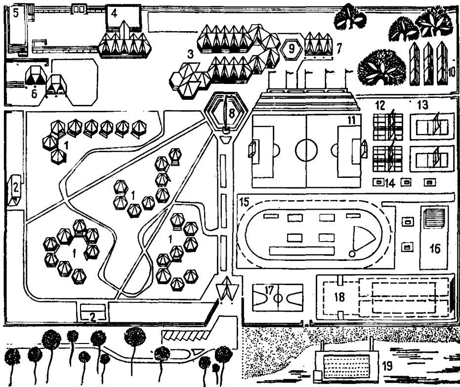
Рис. 35. Пример формирования генерального плана ОЛС на 160 мест из корпусов (табл. 8; рис. 36, 37)
