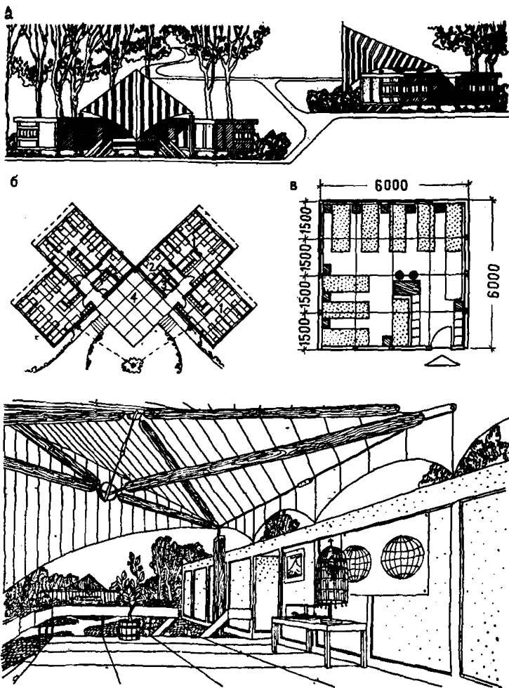
Рис. 11: Спальный корпус на 36—40 чел., технический проект № 169-583 пионерского лагеря с вариантом использования для ОЛС (ЦНИИЭП КТК) a — фасад; б — план корпуса: 1 — спальная комната; 2 — комната педагогов; 3 — подсобная; 4 — веранда; в — схема жилой ячейки; г — интерьер веранды
