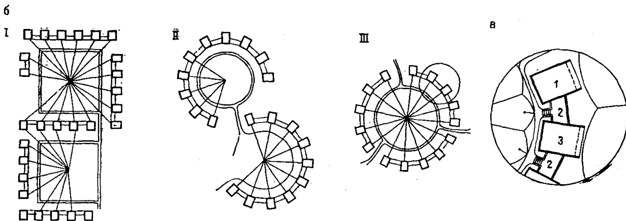
Рис. 13. Спальные павильоны. Экспериментальный проект ОЛС на 400 мест № 1-147 (ЦНИИЭП КТК, архит. Бежанин А. И., Строгий В. А. Фомин К. Д., инж. Липатникова И. Н., Шинман М. Х.)
