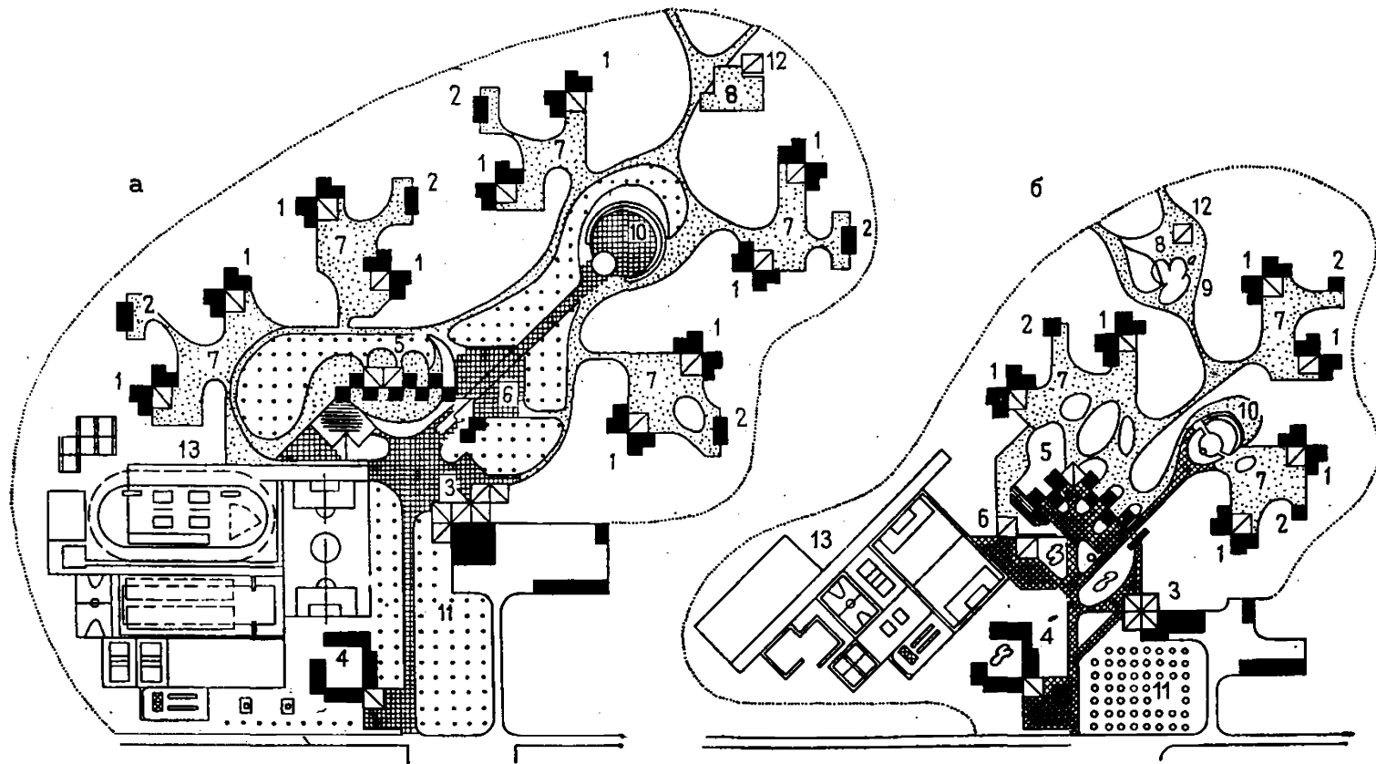
Рис. 3. Схемы генеральных планов пионерских лагерей по техническим проектам № 169-582 (а) и 169-583 (б) с вариантом использования для ОЛС; ЦНИИЭП КТК; архит. Гедулян Е. Н., инженеры Липатникова И. Н., Рябов А. А.
