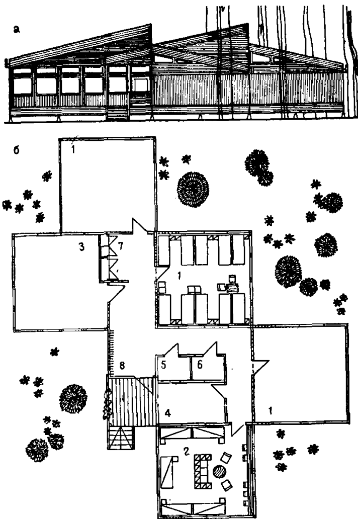
Рис. 12. Спальный корпус на 36—40 чел.; типовый проект № 169-661 пионерского лагеря из щитовых конструкций с вариантом использования для ОЛС (ЦНИИЭП КТК) архитекторы Барышев Д. А., Панкратова О. В., Посвянская Н. А., инженеры Рябов А. А., Сединова В. И.
