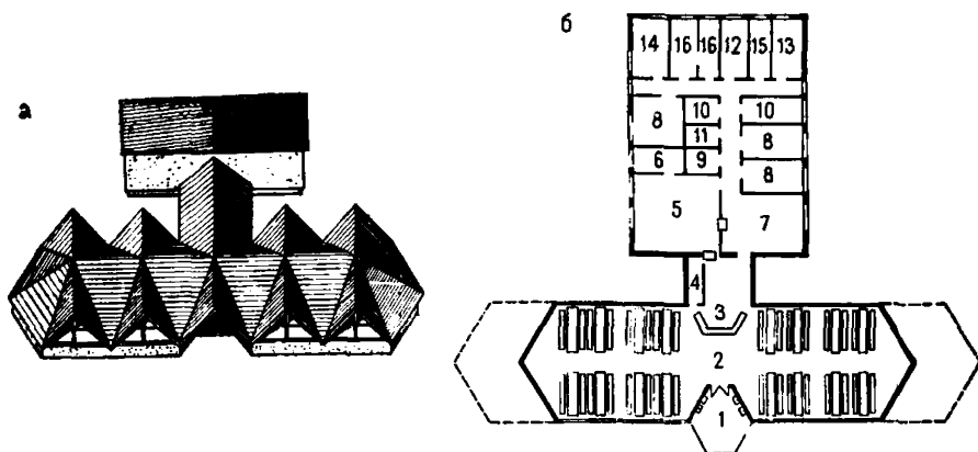
Рис. 36. Корпус столовой оздоровительного лагеря на 160—240 мест (проектное предложение Л. А. Александровой и О. Ф. Коршунова, ЦНИИЭП КТК)
