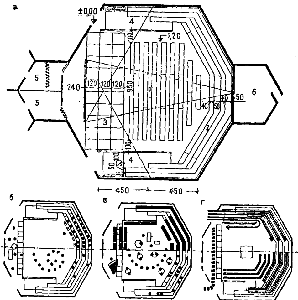
Рис. 19. Схема универсального зала оздоровительного лагеря на 240 мест (предложение Л. А. Александровой, О. Ф. Коршунова; ЦНИИЭП КТК) a — габаритный план с расстановкой оборудования: 1 — центральная часть зала со складывающимися скамьями; 2 — стационарный амфитеатр; 3 — сборно-разборная эстрада; 4 — пандусы; 5 — артистическая комната; 6 — кинопроекционная; б — схема загрузки зала и построения на линейку при проведении лагерного ритуала; в — схема проведения концертов и представлений на сцене-арене, вечеров отдыха с танцами, массовыми играми, аттракционами в кругу; г — схема проведения репетиции кружков народного и бального танца, хора, оркестра, драматической студии и т. п.
