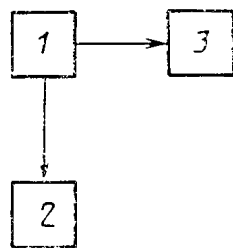
1—образцовая установка К2-38; 2—электронно-счетный частотомер; 3—поверяемый АС
