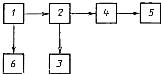
1—генератор ВЧ или СВЧ сигнала; 2—калибратор мощности; 3—мост постоянного тока; 4—согласующий аттенуатор; 5—поверяемый АС; 6—электронно-счетный частотомер
