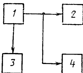
1—генератор гармонических сигналов; 2—поверяемый АС; 3—электронно-счетный частотомер; 4—измеритель уровня.
