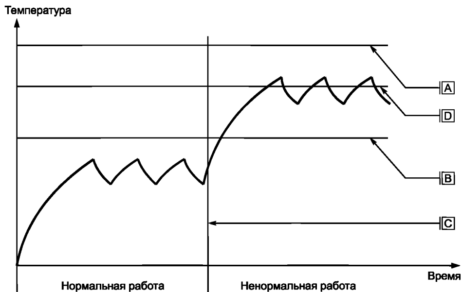
Рисунок ЕЕ.4 — Термовыключатель с самовозвратом
