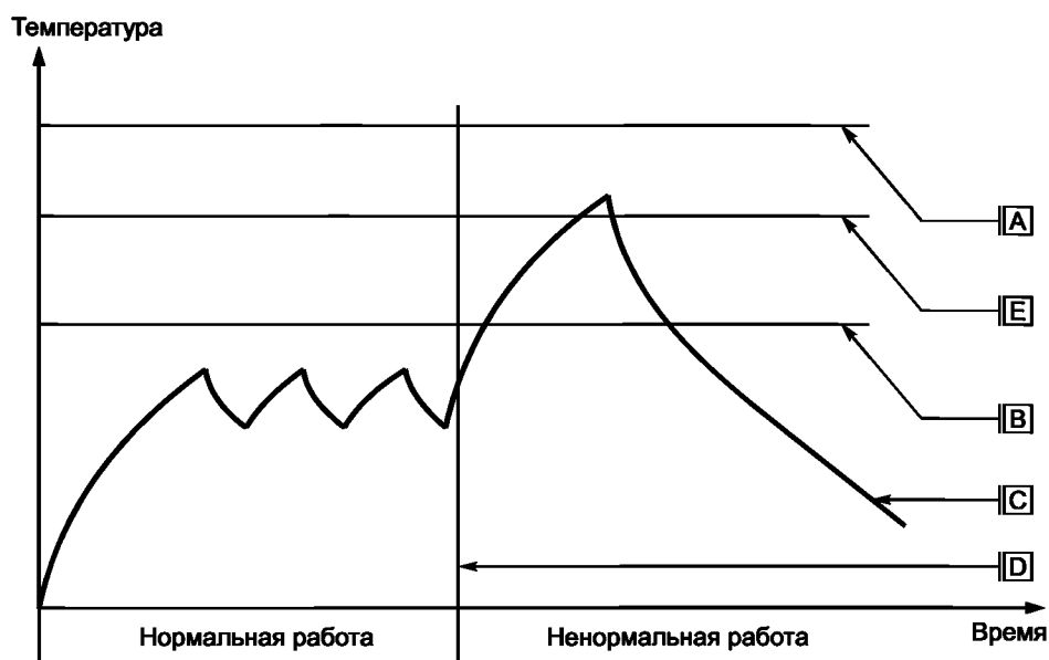
Рисунок ЕЕ.4 — Термовыключатель с самовозвратом
