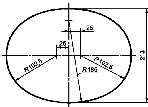
Рисунок 3 — Размеры отверстия в основании термокамеры
