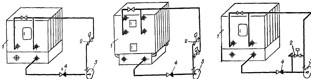
Рис. 14. Обвязка камеры орошения а — вариант 1; б — вариант 2; в — вариант 3; 1 — камера орошения; 2 — регулирующий клапан; 3 — насос; 4 — обратный клапан
