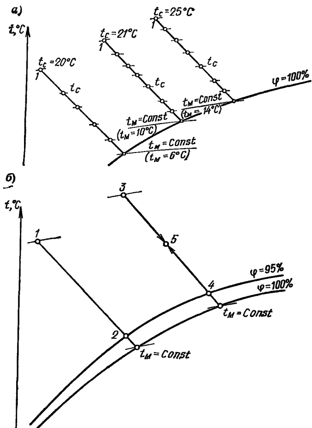
Рис. 2. Конечные параметры воздуха после смесительных контактных аппаратов
