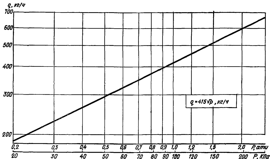
Рис. 7. Расходная характеристика широкофакельных форсунок ШФ 5/9 q = 415\sqrt{P} , кг/ч, где k=415 — расходный коэффициент, P — давление перед форсунками, атм
