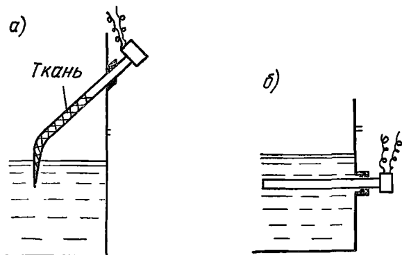
Рис. 9. Варианты установки датчика температуры мокрого термометра
