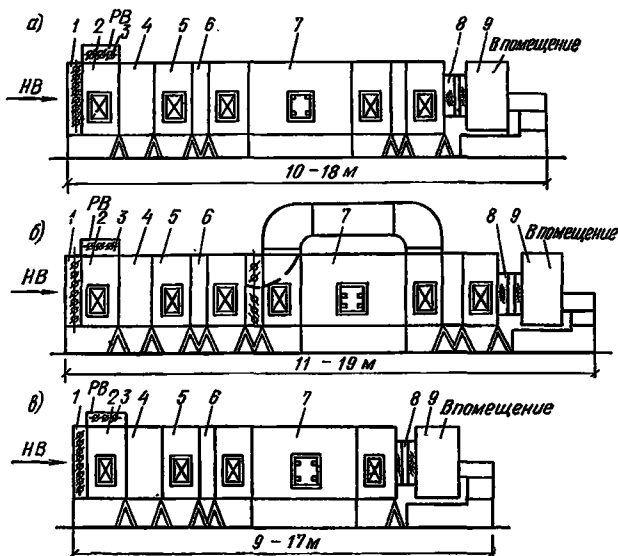
Рис. 1. Технологические схемы центральных однозональных кондиционеров
