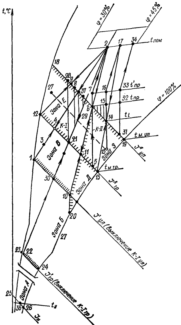
Рис. 4. Сравнение на t-d -диаграмме режимов работы систем кондиционирования воздуха с рециркуляцией: УПА и традиционной:
