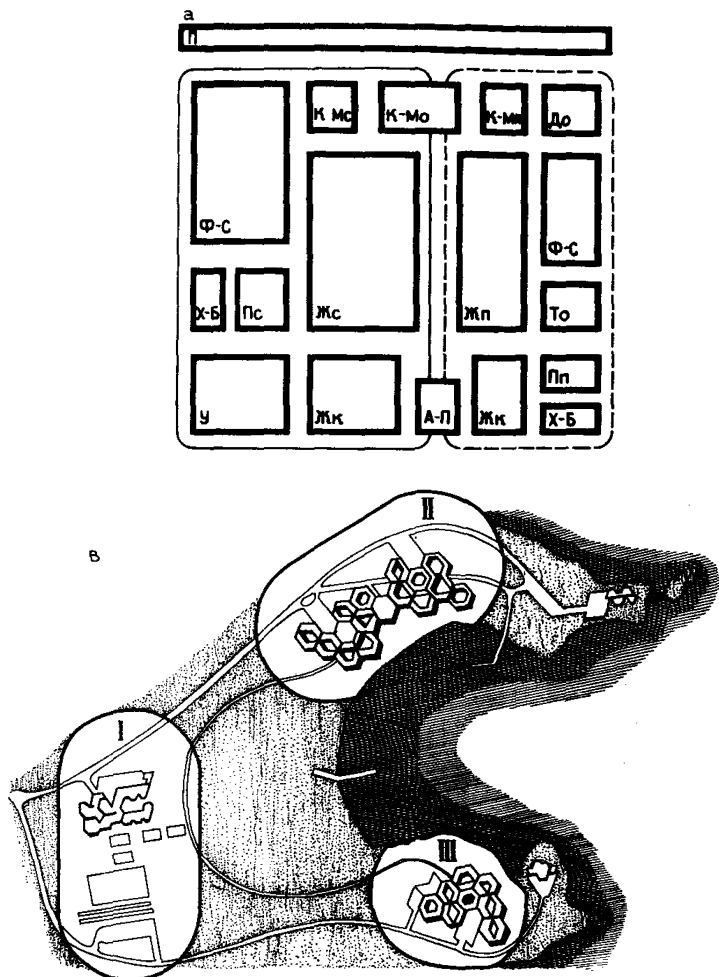
Рис. 8. Примеры решения генеральных планов БОВК с разделным проживанием студентов и преподавателей вузов и полной централизацией средств обслуживания
