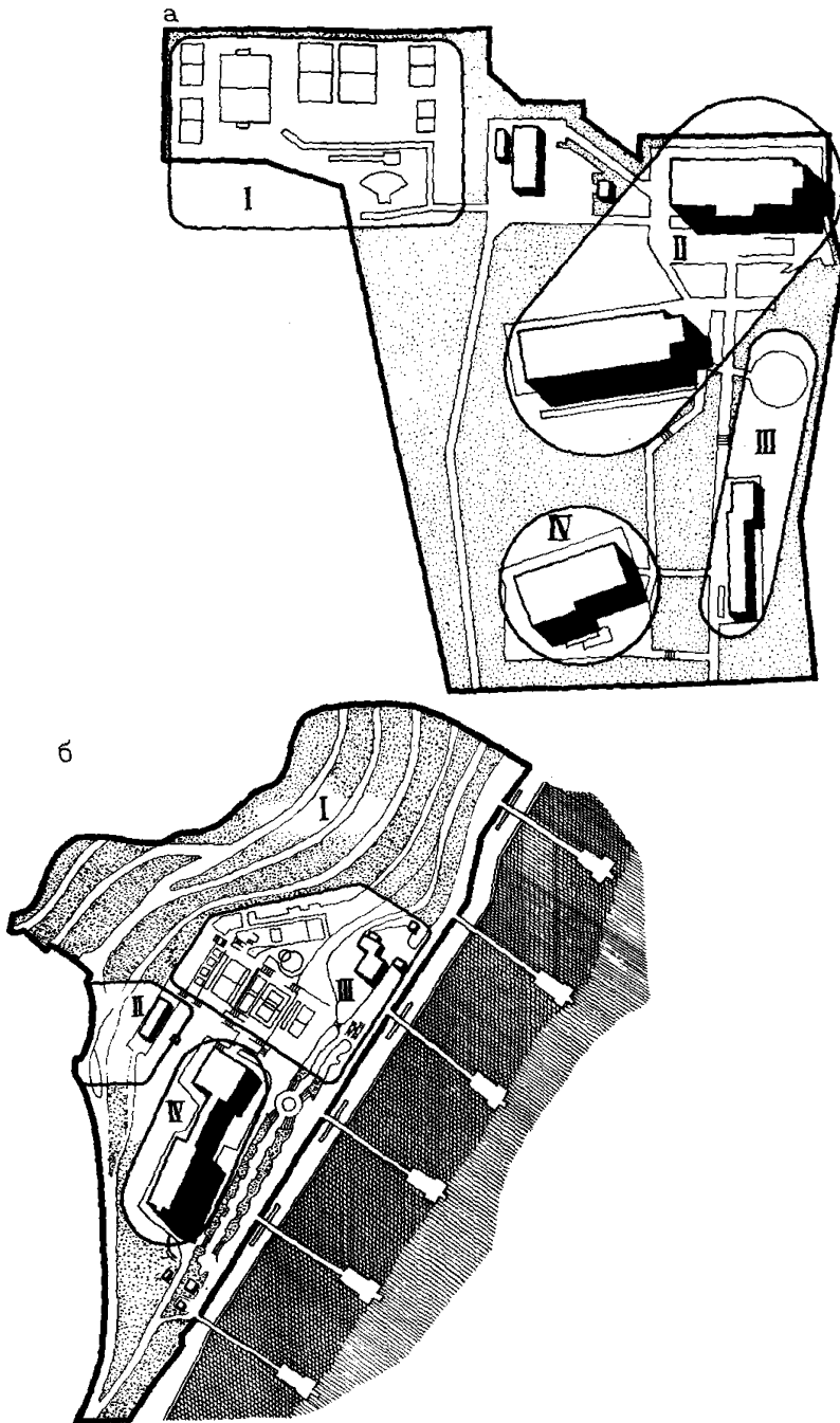
Рис. 6. Примеры решения генеральных планов БОВК с совместным проживанием студентов и преподавателей вузов а – база отдыха Харьковского авиационного института на 400 мест в пос. Рыбачье, Крым; I – спортивная зона; II – жилая зона студентов и преподавателей; III – зоны культмассового обслуживания; IV – зона питания; б – база отдыха Московского авиационного института на 500 мест в г. Алуште, Крым; I – места для палаток; II – хозяйственная зона; III – зона спортивного и культмассового обслуживания; IV – жилая зона студентов и преподавателей
