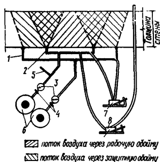
Рис. 12. Схема установки для испытания стены на воздухопроницаемость
