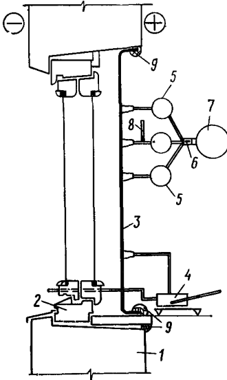
Рис. 11. Схема установки для испытания окна на воздухопроницаемость
