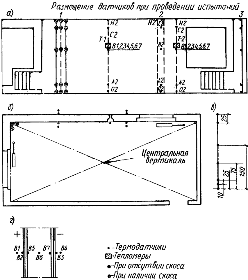
Рис. 1. Размещение датчиков при проведении испытаний а — развертка стен; б — план помещения; в — центральная вертикаль; г — сечение стены; 1 — наружный угол; 2 — стык наружных панелей; 3 — стык наружных и внутренней панелей; термопара или термометр B_1 измеряет температуру внутреннего воздуха; B_4 — наружного воздуха; B_2 — внутренней поверхности ограждения, B_3 — наружной поверхности ограждения
