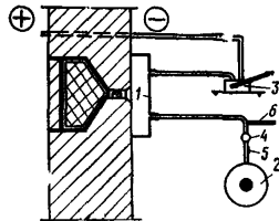
Рис. 10. Схема установки для испытания заделки устья стыка на воздухопроницаемость 1 — металлическая обойма; 2 — источник разрежения (пылесос); 3 — микроманометр; 4 — измеритель расхода воздуха; 5 — шибер или газовый кран; 6 — термометр
