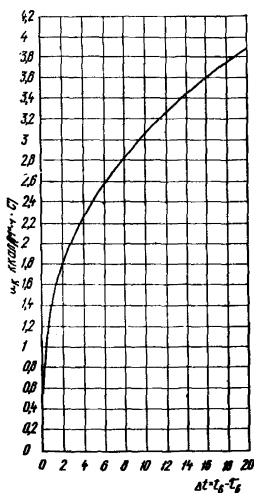
Рис. 4. График для определения \alpha_k
