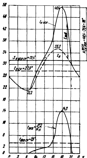
Рис. 9. Графическое определение амплитуды колебания температуры наружного воздуха с учетом солнечной радиации A_{\text{сол}} экв. t_{\text{вн,ср}} .
