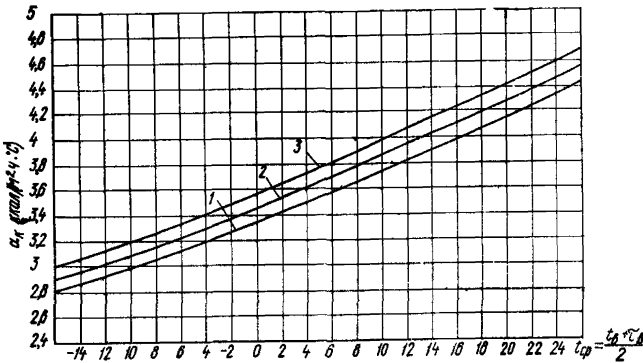
Рис. 5. График для определения \alpha_l
