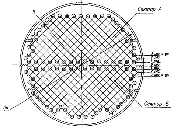
Для перегородок аппаратов диаметром от 400 до 1200 мм
