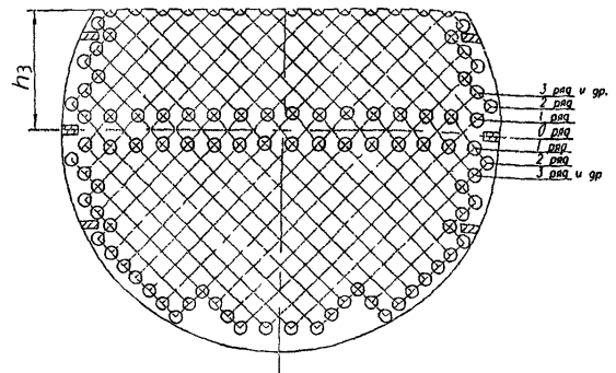
Для перегородок аппаратов диаметром от 400 до 1200 мм
