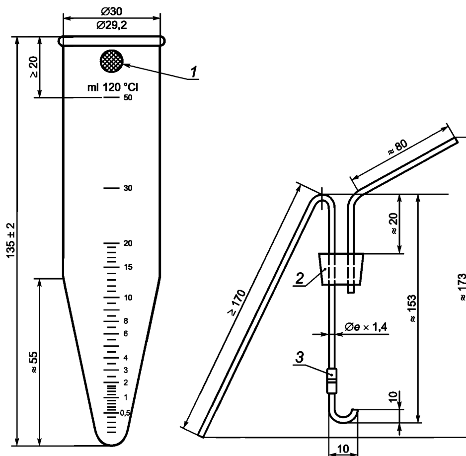
1 — матовая поверхность; 2 — резиновая пробка; 3 — гибкая пластмассовая трубка
