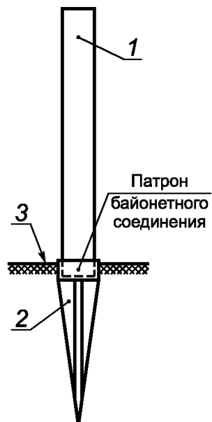
1 — корпус столбика; 2 — удерживающее устройство; 3 — поверхность грунта
