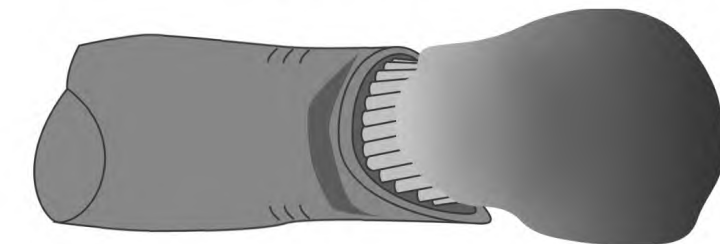
б) Чрезмерное лужение провода
