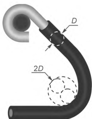
Рисунок 11 — Снятие напряжения с проволочного вывода: допустимое состояние
