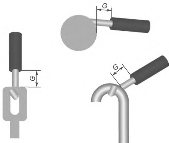
Рисунок 12 — Оценка зазора изоляции: допустимое состояние
