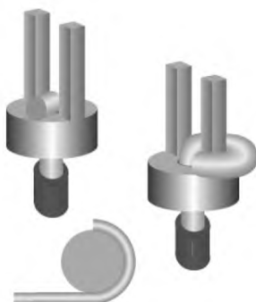
Рисунок 9 — Соединение контакта с нижней разводкой: допустимое состояние
