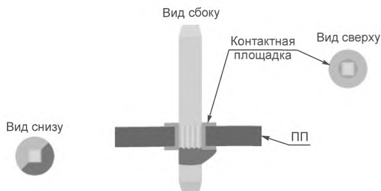
Рисунок 19 — Галтели припоя: допустимое состояние
