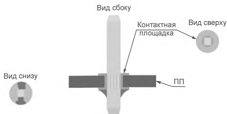
Рисунок 20 — Галтели припоя: недопустимое состояние
