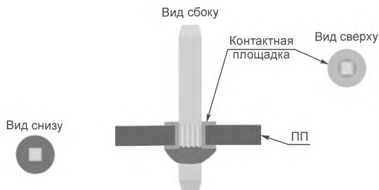
Рисунок 18 — Галтели припоя: допустимое состояние
