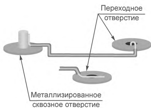
Рисунок 30 — Соединение навесной перемычки с выступающими выводами компонентов и металлизированными отверстиями: виды состояний
