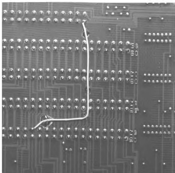
Рисунок 28 — Прикрепление провода: допустимое состояние
