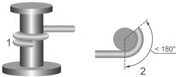
Рисунок 4 — Круговая накрутка провода и вывода: виды состояний
