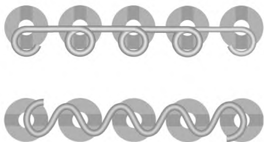
Рисунок 10 — Непрерывная прокладка шины: допустимое состояние
