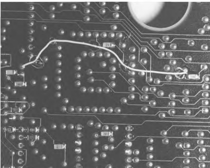
Рисунок 26 — Прокладка провода около контактных площадок: виды состояний
