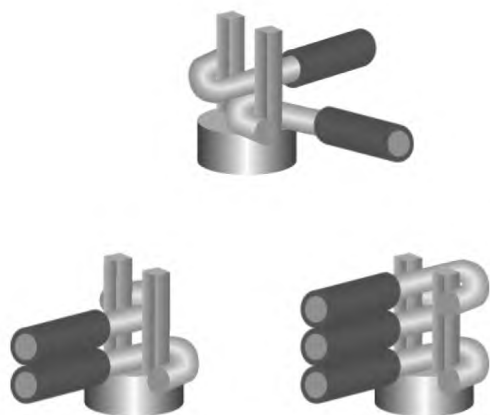
Рисунок 6 — Боковое соединение разводки, вилкообразный контакт: допустимое состояние
