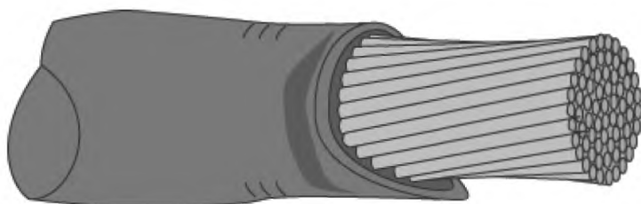
Рисунок 14 — Поврежденная изоляция: допустимое состояние
