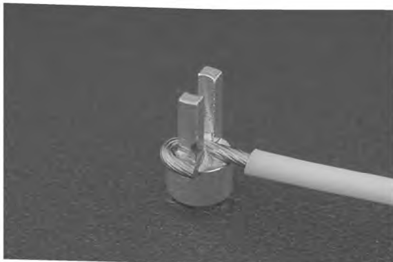
Рисунок 35 — Паяное соединение провода с контактом: допустимое состояние
