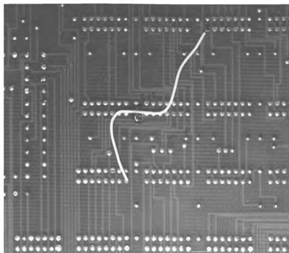
Рисунок 29 — Незакрепленный провод: виды состояний
