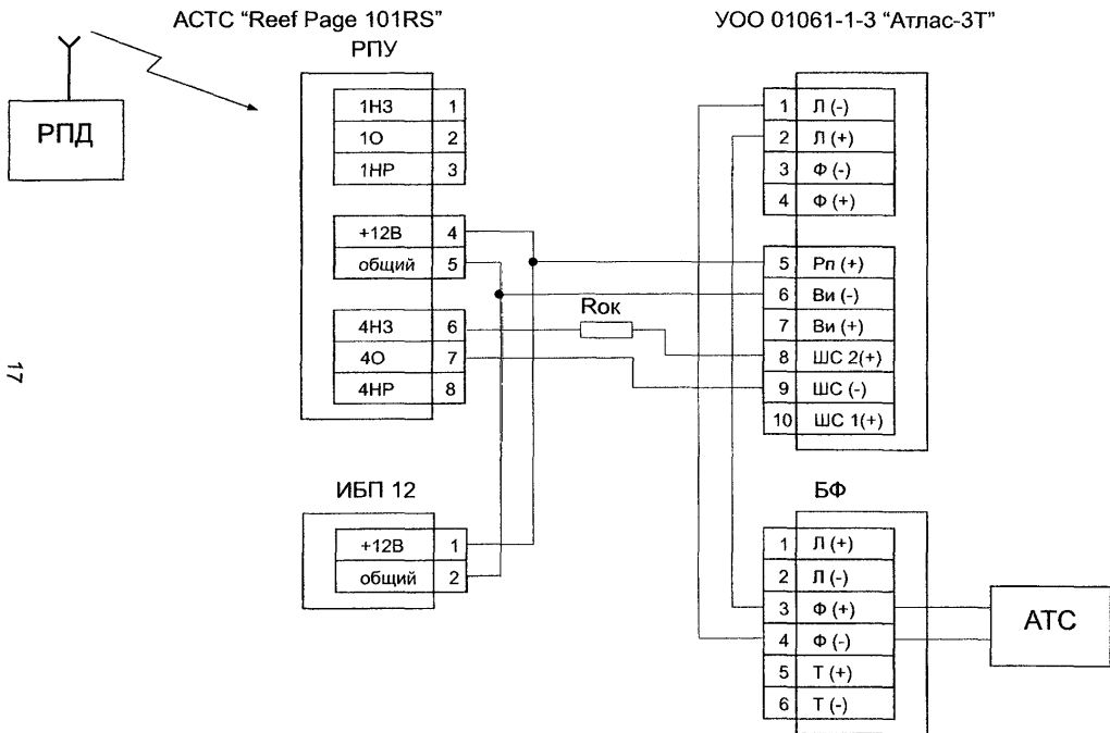
Рис 6 - Схема подключения АТС "Reef Page 101RS" к УОО 01061-1-3 "Атлас-3Т"
