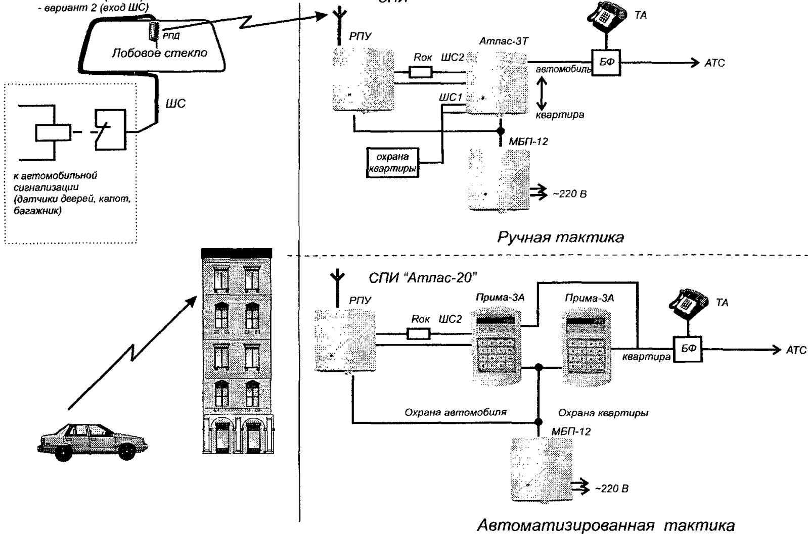
Рис. 5 - Схема подключения РТС "Радиокнопка" к СПИ "Атлас-20"
