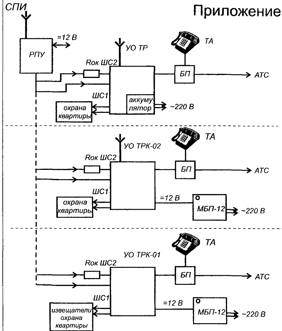
Рис. 1 - Схема подключения РТС "Радиокнопка" к СПИ "Фобос-ТР", "Фобос-3"
