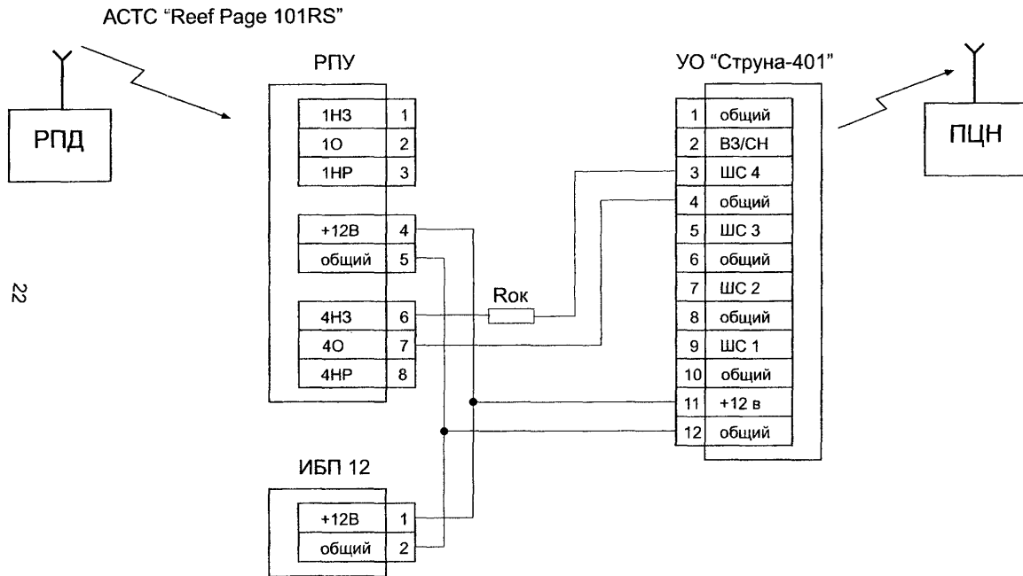
Рис 11 - Схема подключения ACTC "Reef Page 101RS" к УО "Струна-401"
