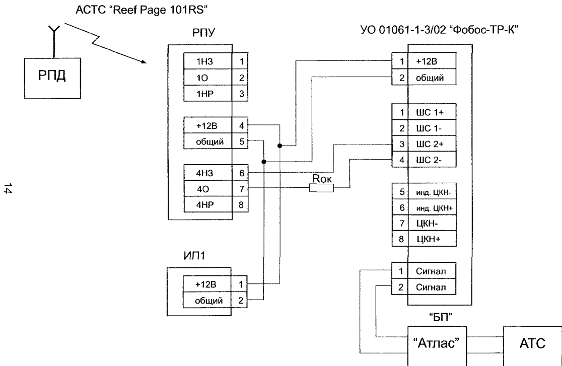
Рис. 3 - Схема подключения АТС "Reef Page 101RS" к УО 01061-1-3/02 "Фобос-ТР-К"
