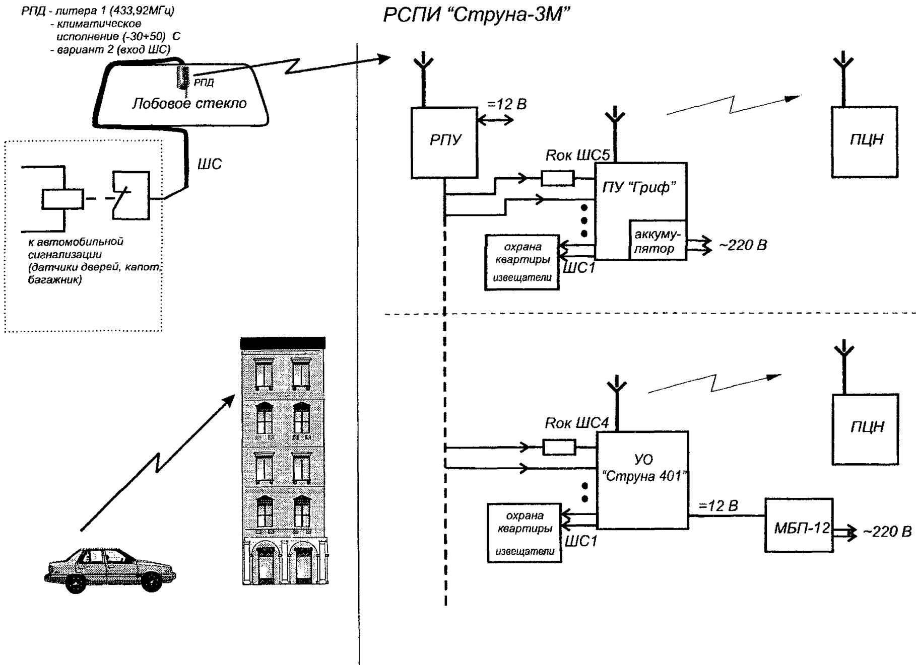
Рис. 9 - Схема подключения РТС "Радиокнопка" к РСПИ "Струна-3М"
