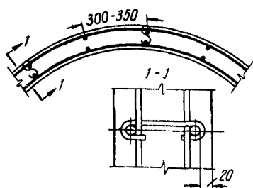
Рис. 6. Стена силоса с двойной арматурой
