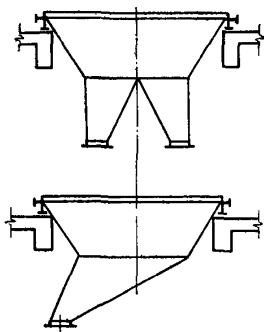
Рис. 12. Воронки днищ силосов с выпусками, смещенными относительно оси силоса
