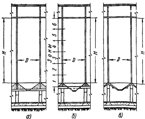
Рис. 1. Разрезы силосов
