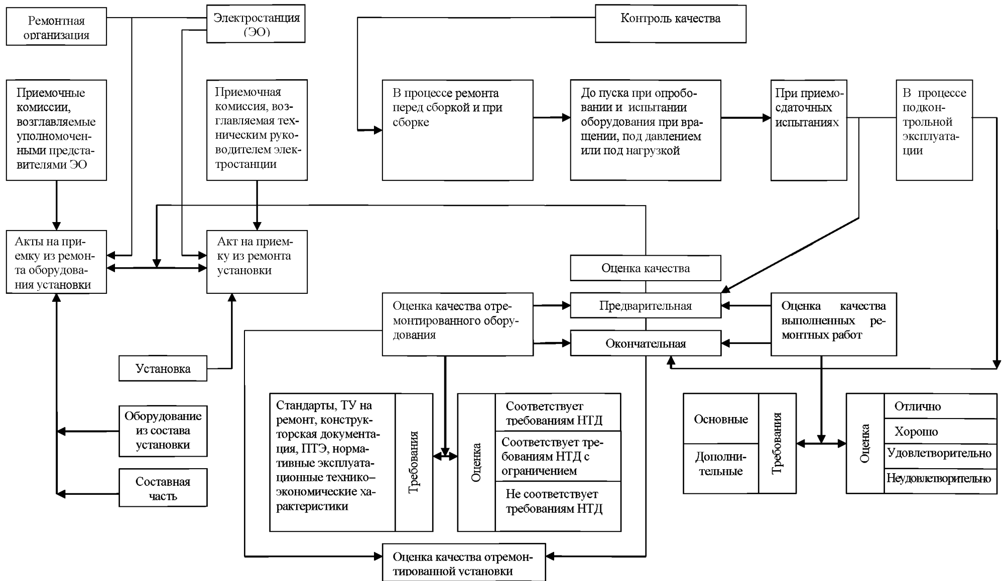
Рисунок 1 – Принципиальная схема оценки качества ремонта
