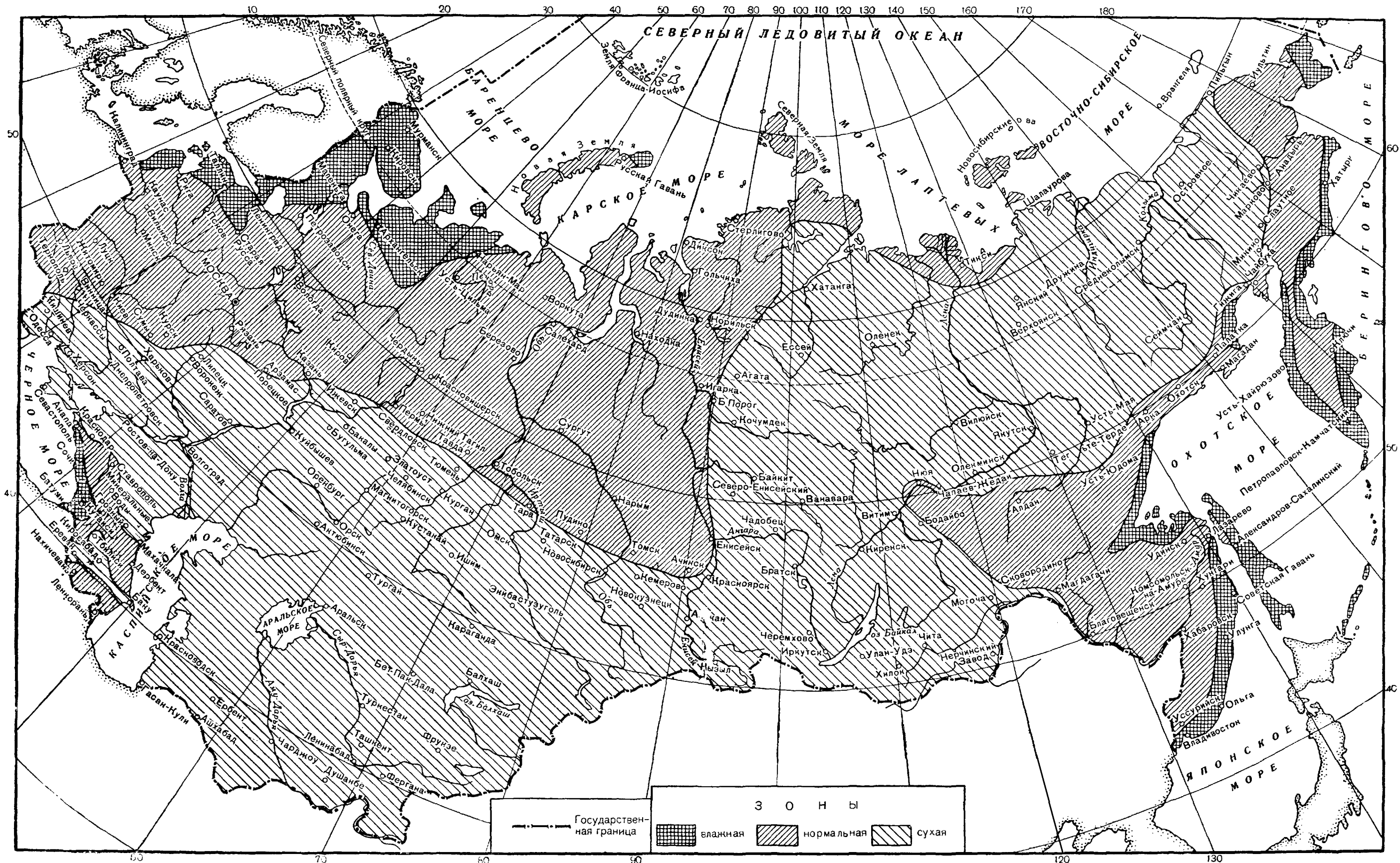
Рис. 1. Схематическая карта территории СССР для назначения коэффициентов теплопроводности материалов ограждающих конструкций зданий
