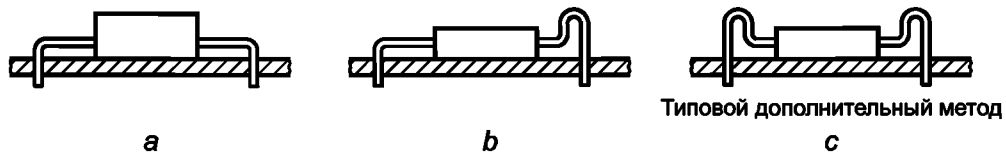
Рисунок А.8 — Примеры формы выводов
