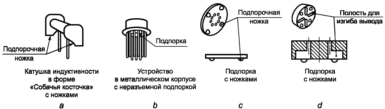
Рисунок А.6 — Монтаж с упорами и подпорками
