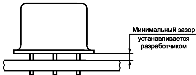
Рисунок А.1 — Монтаж свободно стоящих компонентов
