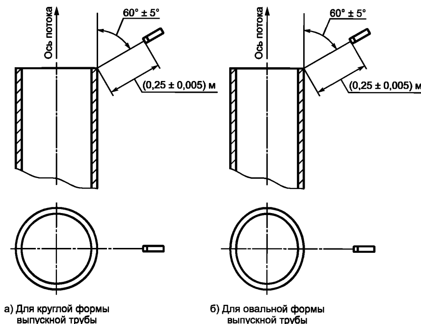
Рисунок 6 — Расположение микрофона для измерения шума процесса выпуска
