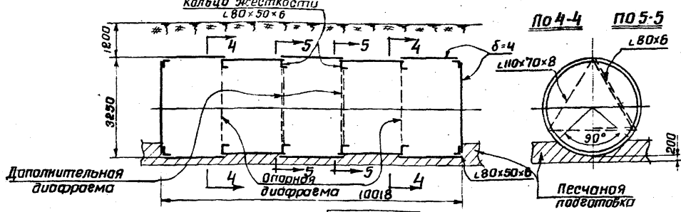
Резервуары 100 3 м 3 704-1-48 (200 п) 704-1-48 (200 р п)
