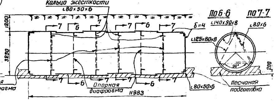
Резервуары 100 3 м 3 704-1-48 (200 п) 704-1-48 (200 р п)
