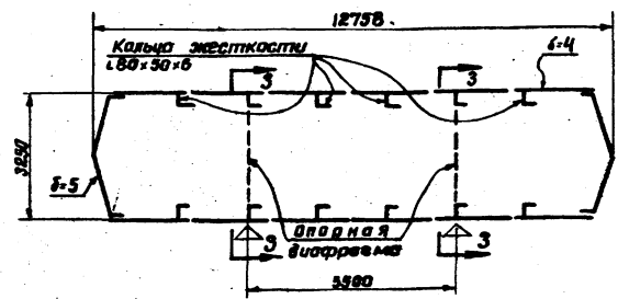
Резервуар 100м³ N 704-1-48(КА 200/20)
