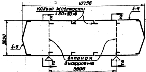
Резервуар 100м³ N 704-1-48(КА 200/20)
