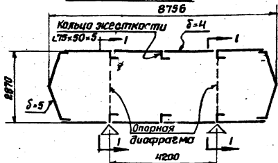
Резервуар 75м³ N 704-1-47(КА 200/20)
