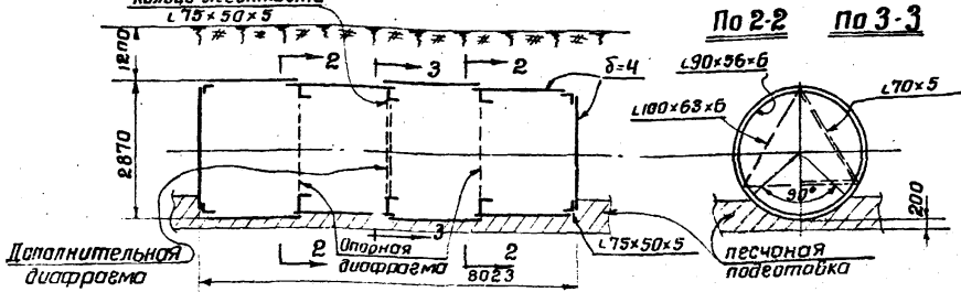
Резервуары 75 3 м 3 704-1-47 (200 п) 704-1-47 (200 р п)
