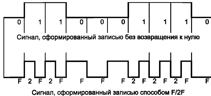
Рисунок В.1 — Кодирование F/2F
