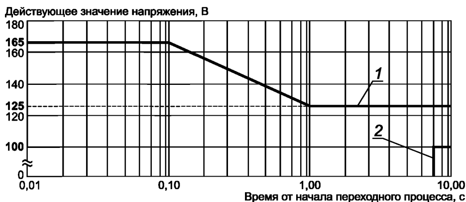
Рисунок 7 — Пределы ненормальных повышенных и пониженных напряжений переменного тока постоянной частоты 400 Гц
