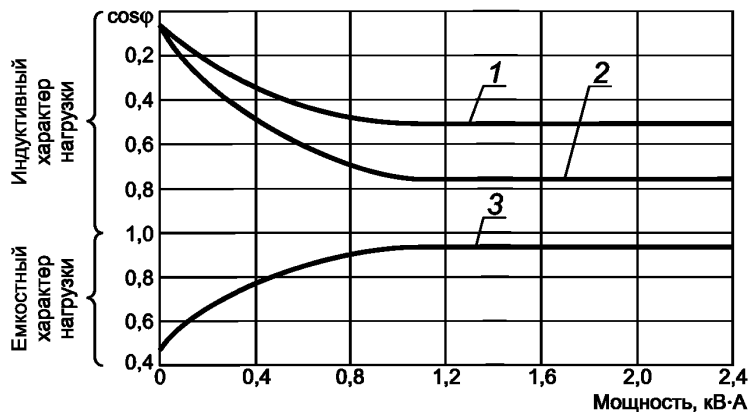
Рисунок 17 — Пределы значений коэффициента мощности приемника
