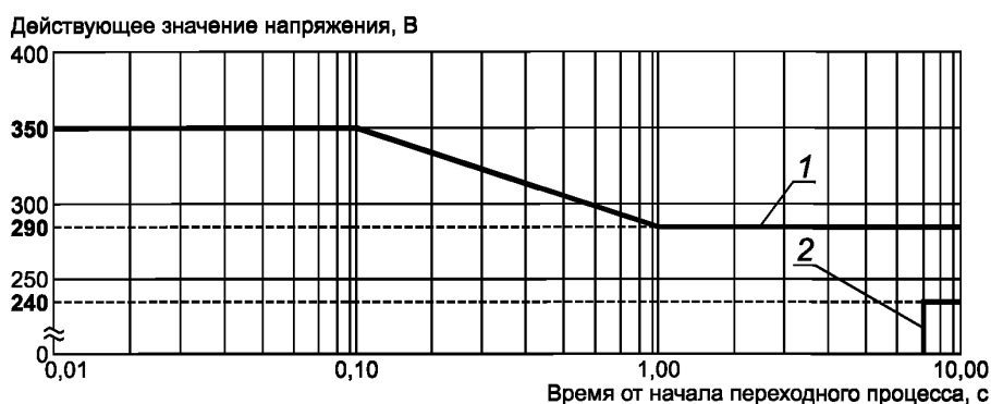
Рисунок 15 — Пределы ненормальных повышенных и пониженных напряжений систем постоянного тока 270 В
