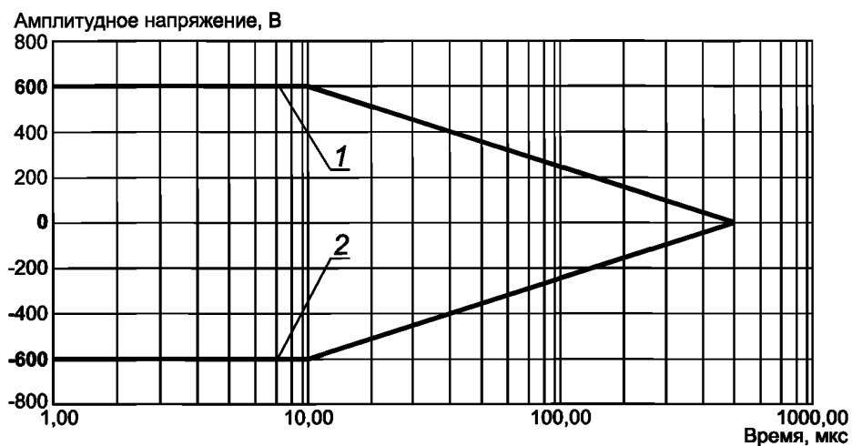
Рисунок 18 — Огибающая импульсов напряжения для приемников постоянного и переменного токов
