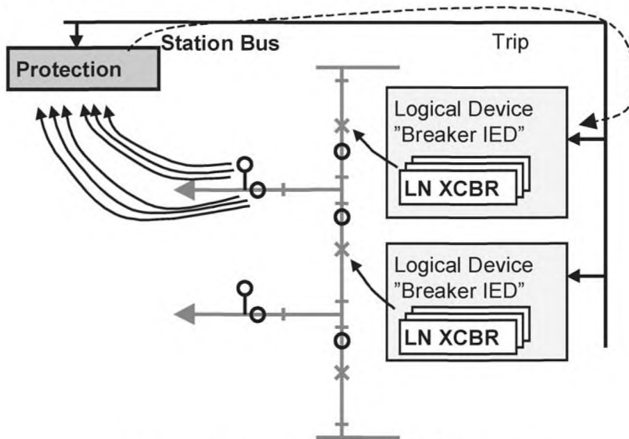
Рисунок 4 — Принцип построения устройств, лист 1
