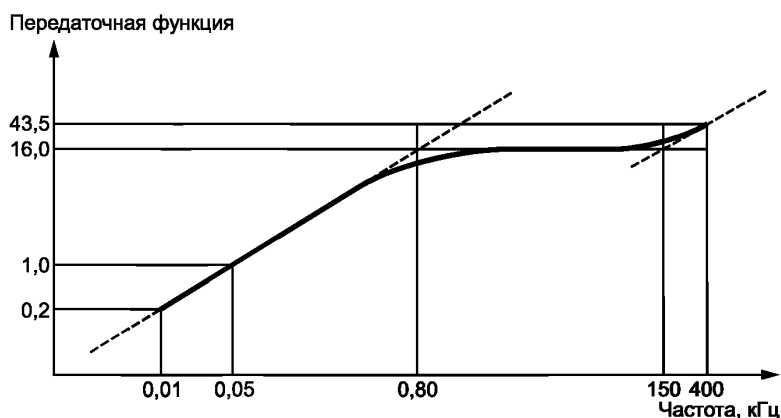
Рисунок 1 — Передаточная функция
