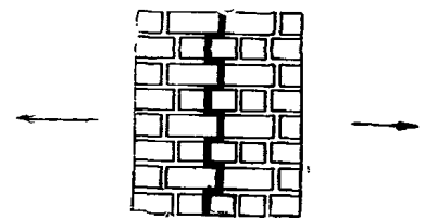
Рис. 2. Растяжение кладки по перевязанному сечению
