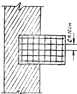
Рис. 5. Железобетонные распределительные плиты
