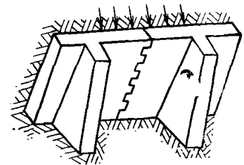
Рис. 3. Растяжение кладки при изгибе по перевязанному сечению
