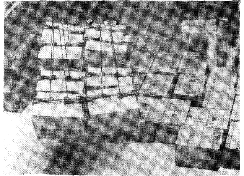
Рис.205.6. Формирование в просвете люка тричного штабеля целлюлозы с помощью крана, оснащенного комплектом подвесок с захватами. Порт Таллин.
