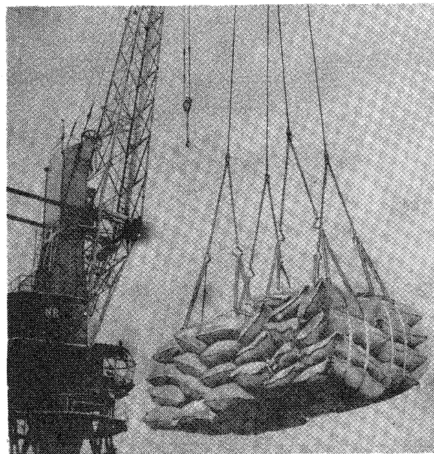
Рис.103.4. Крановый "подъем" при погрузке в судно пакетов муки в стропах для пакетирования. Порт Калининград.
