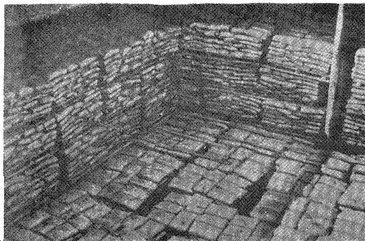
Рис. I06.11. Размещение пакетов груза на поддонах в просвете люка и в подпалубном пространстве трюма. Порт Керчь.
