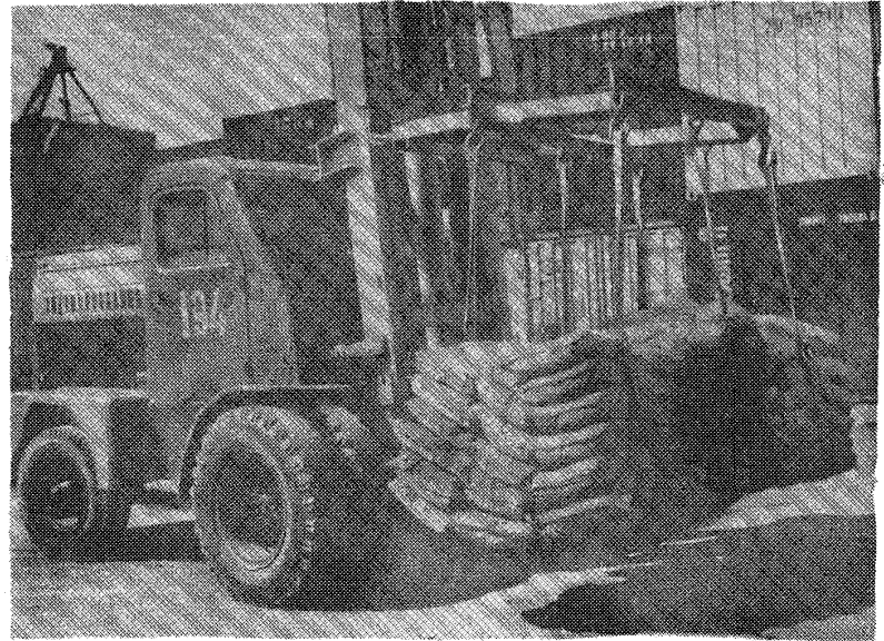
Рис.106.2. Внутрипортовое транспортирование пакетов цемента (в стропках для пакетирования) погрузчиком, оборудованным рамой с комплектом 2-х краевых подвесок. Порт Владивосток.
