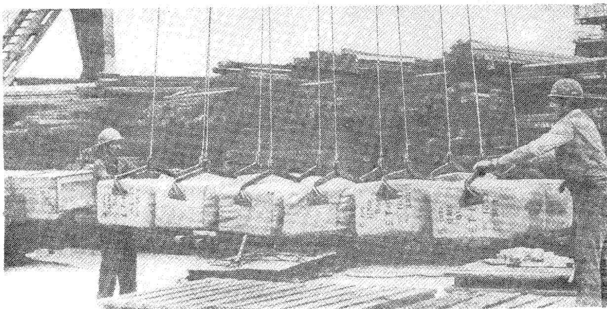
Рис.203.2. Выгрузка из судна на причал табака в кипах краном, оснащенным рамой и комплектом подвесок с захватами. Порт Измаил.
