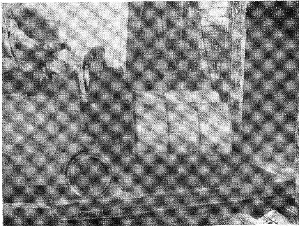
Рис.303.5. Погрузка в крытый вагон бочек погрузчиком, оборудованным многовилочным захватом (типа УЗНС-1). Порт Ленинград.
