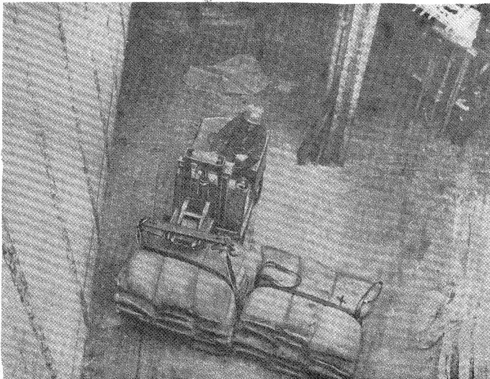
Рис.103.5. Транспортирование в подпалубное пространство пакетов муки (в стропах для пакетирования) погрузчиком, оборудованным крюковой подвеской. Порт Владивосток.
