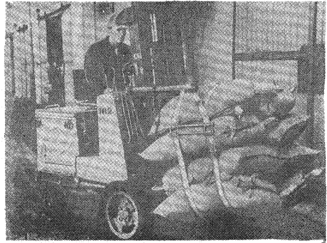
Рис.103.2. "Подъем" погрузчика, оборудованного двухтыревым захватом при перевозке пакетов шрота в стропах для пакетирования. Порт Ленинград.
