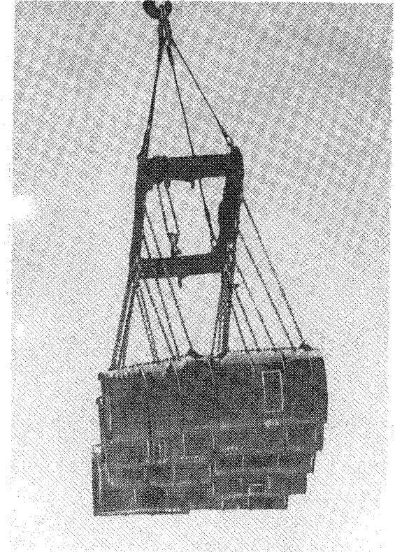
Рис.303.4. Перегрузка бочек краном, оснащенный рамой с комплектом храпов. Порт Вентспилс.
