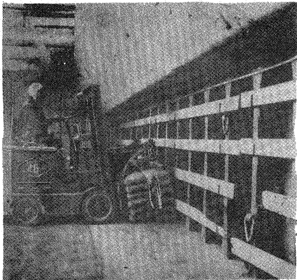
Рис. I06.10. Установка в подпалубном пространстве пакетов цемента (в стропях для пакетирования) погрузчиком, оборудованным комплектом 2-х крюковых подвесок. Порт Владивосток.
