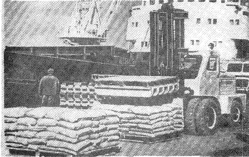
Рис.106.5. Кантование груза с плоского поддона на гребенчатый погрузчик, оборудованным захватом-кантователем. Порт Керчь.
