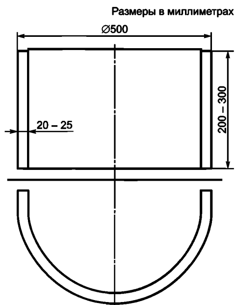
Рисунок 3 — Центробежнолитая трубная заготовка для изготовления СО СФФ
