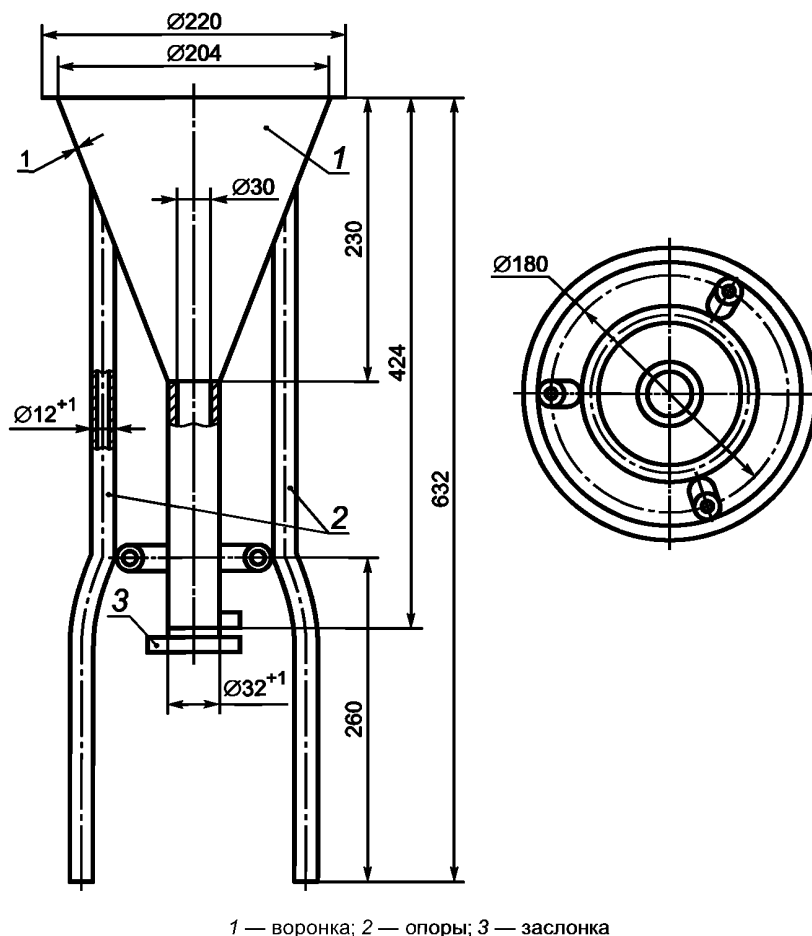
1 — воронка; 2 — опоры; 3 — заслонка
