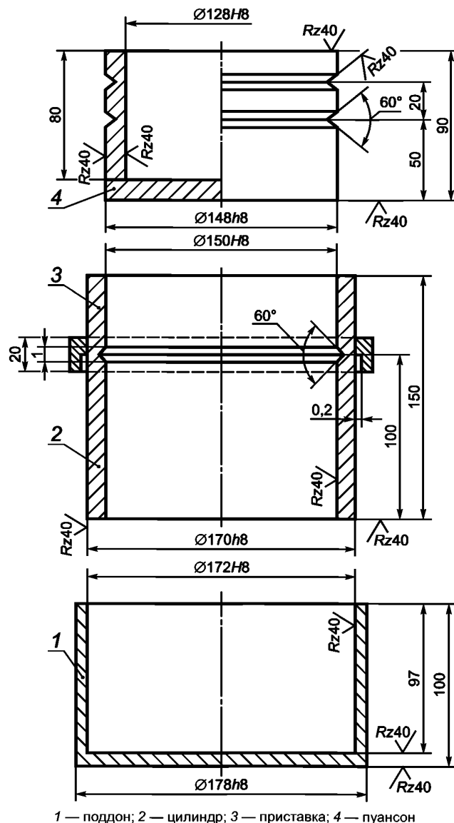
1 — поддон; 2 — цилиндр; 3 — приставка; 4 — пуансон
