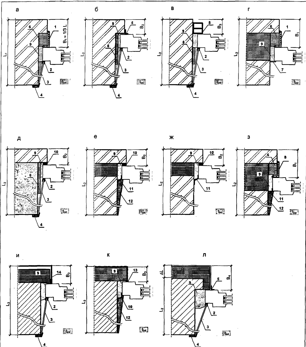
Рис.7.1. Основные варианты узлов примыкания оконных блоков к наружным стенам различного конструктивного решения: а, б, в, г – с применением профильных изделий из ПВХ; д, е, ж, з – с применением изоляционных саморасширяющихся и пароизоляционных лент; и, к, л – в наружных стенах с фасадной теплоизоляцией (1 – уголкового профиля; 2 – стартовый профиль; 3 – облицовочная панель из ПВХ; 4 – откосная система профилей; 5 – уголок из ПВХ; 6 – термовкладыш; 7 – нащельник из ПВХ или пароизоляционная лента; 8 – доборный профиль; 9 – пенный утеплитель; 10 – изоляционная саморасширяющаяся паропроницаемая лента или герметизирующая мастика; 11 – пароизоляционная лента; 12 – штукатурка; 13 – атмосферостойкий герметик; 14 – элемент вентилируемой фасадной системы)
