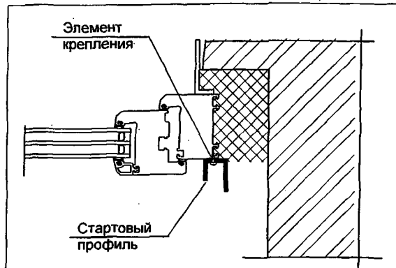
Схема крепления стартовых профилей
