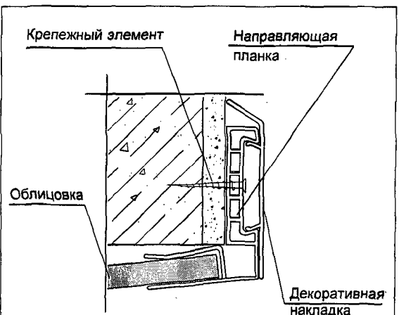
Схема крепления листов облицовки в профилях откосной системы
