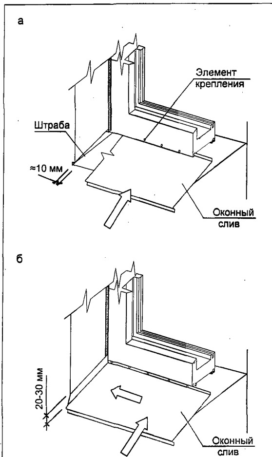
Установка оконного слива: а – вариант с заведением слива в штрабу оконного откоса; б – при отгибе бокового участка оконного слива в месте примыкания к стене
