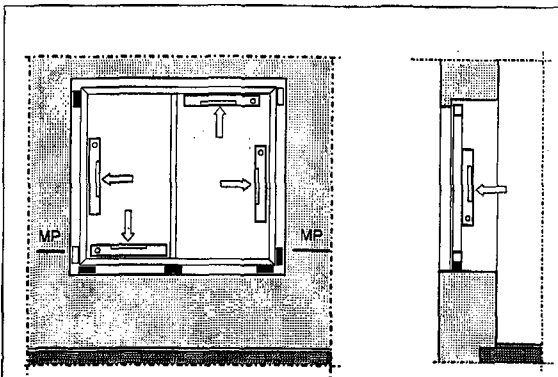
Схема проверки вертикальности установки оконного блока
