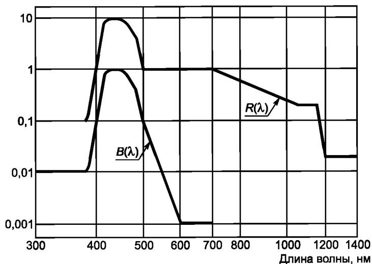
Рисунок 6 — Функция тепловой опасности клетчатки R(\lambda) и функция светлого-голубой опасности клетчатки B(\lambda)
