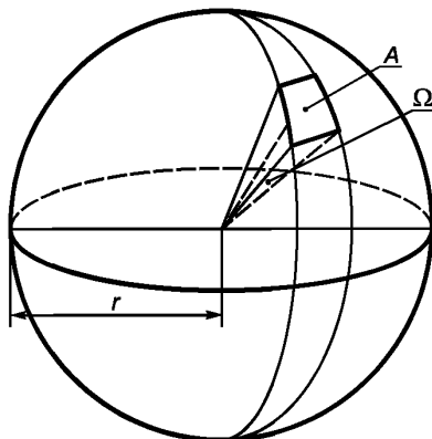
Рисунок 3 — Определение телесного угла
