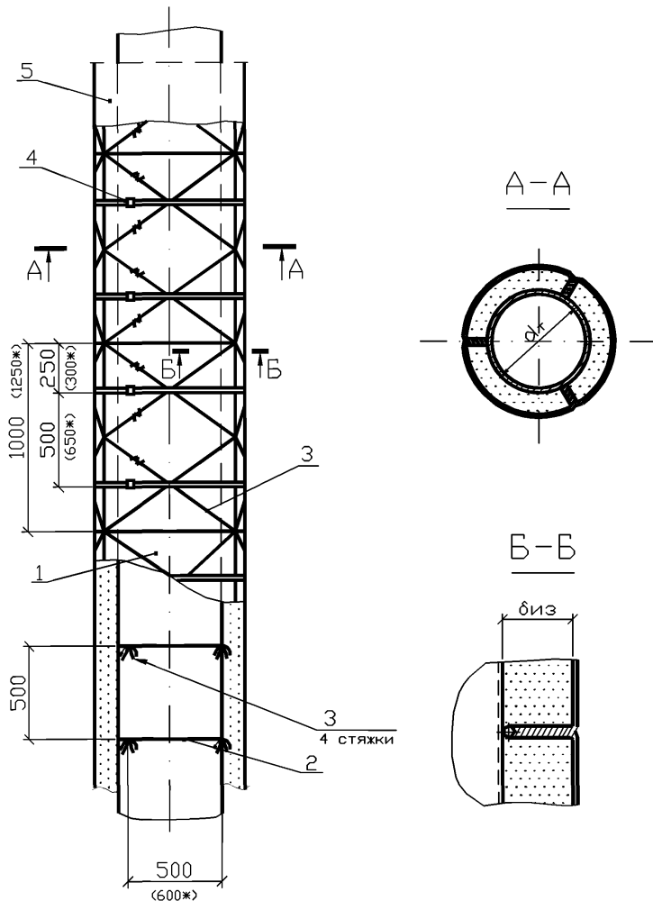
Рис. 8.5 Изоляция трубопроводов наружным диаметром 530 мм и более теплоизоляционными изделиями URSA® в один слой с креплением проволочными стяжками и бандажами
