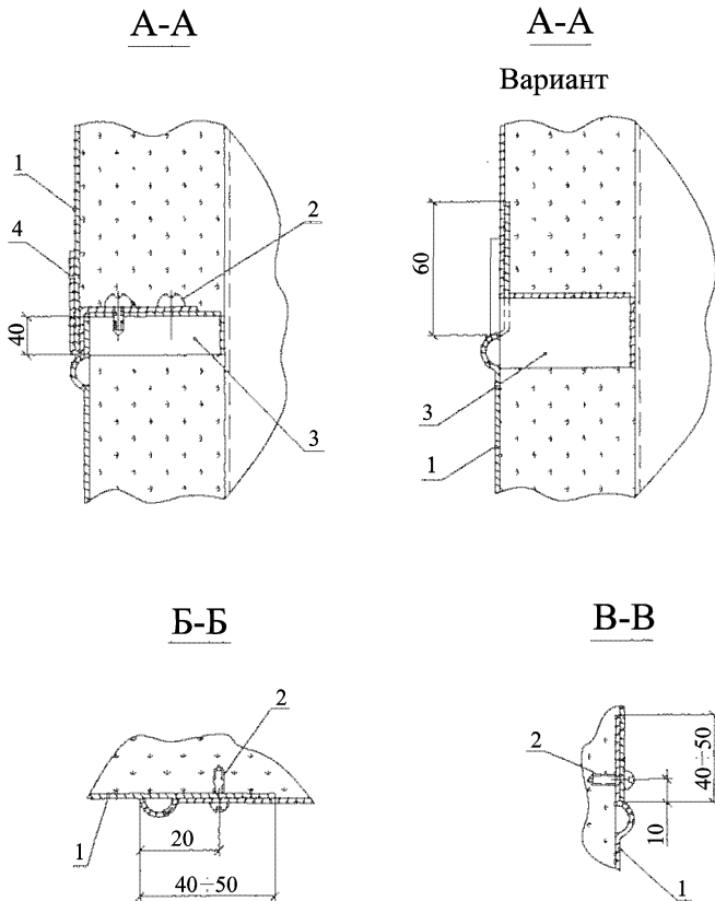
Рис. 4.14 Разрезы А-А и В-В к рис. 4.13
