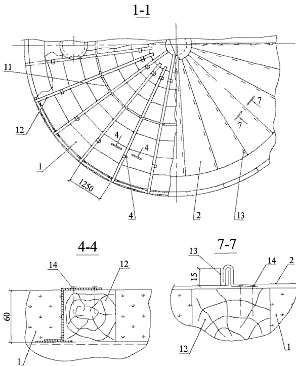
Рис. 4.22 Разрезы 1-1, 4-4, 7-7 к рис.4.21
