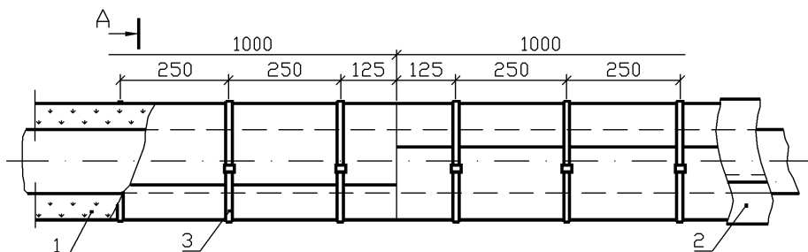
Рис. 8.2 Изоляция трубопроводов наружным диаметром от 57 до 159 мм включительно теплоизоляционными матами URSA®.
