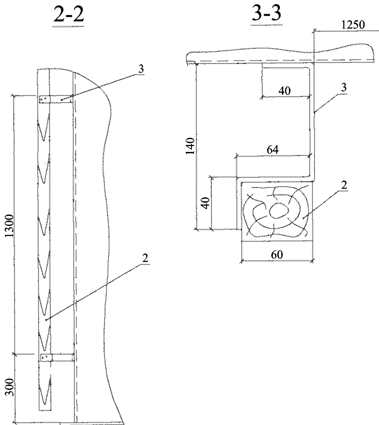
Рис. 4.27 Разрезы 2-2 и 3-3 к рис.4.25
