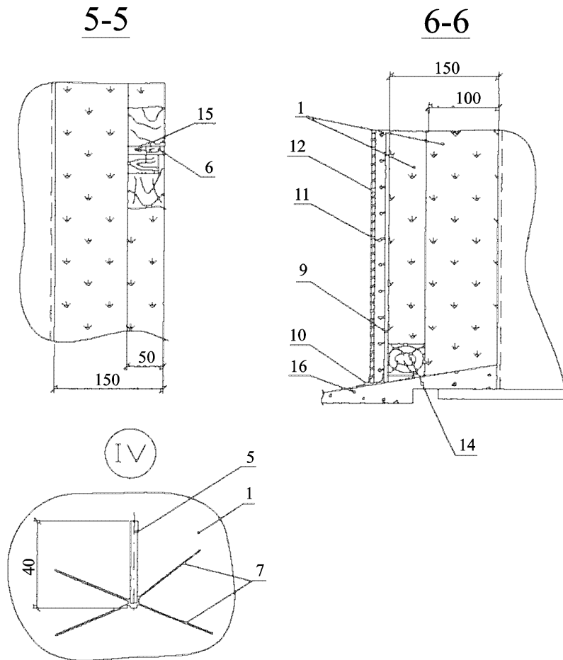
Рис. 4.28 Узел IV и разрезы 5-5 и 6-6 к рис.4.25
