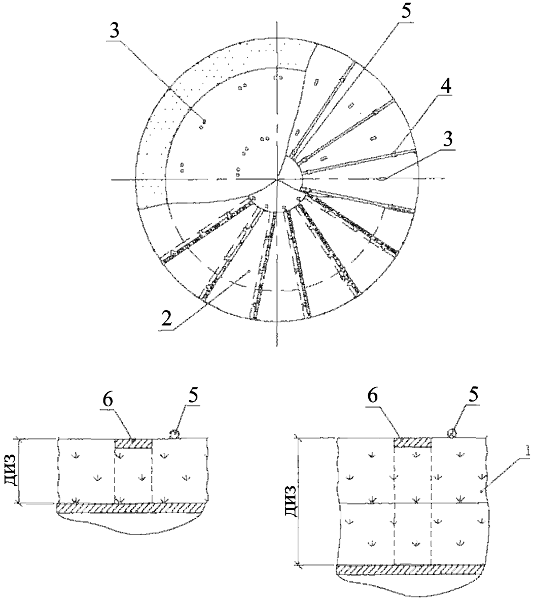
Рис. 4.10 Разрез А-А и узел I к рис. 4.9
