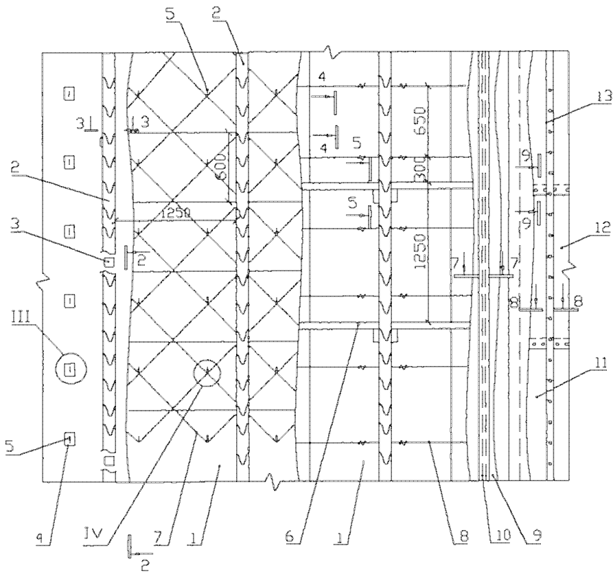
Рис. 4.25 Узел I к рис.4.24. Конструкция тепловой изоляции цилиндрической стенки резервуара
