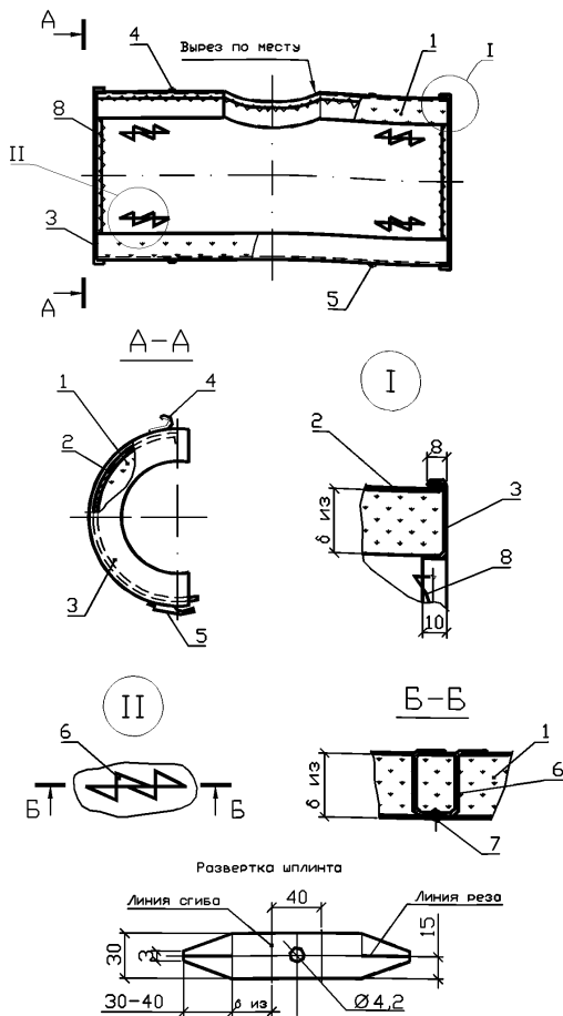
Рис. 8.13 Полуфутляр с вкладышем-матрацем из матов теплоизоляционных URSA®
