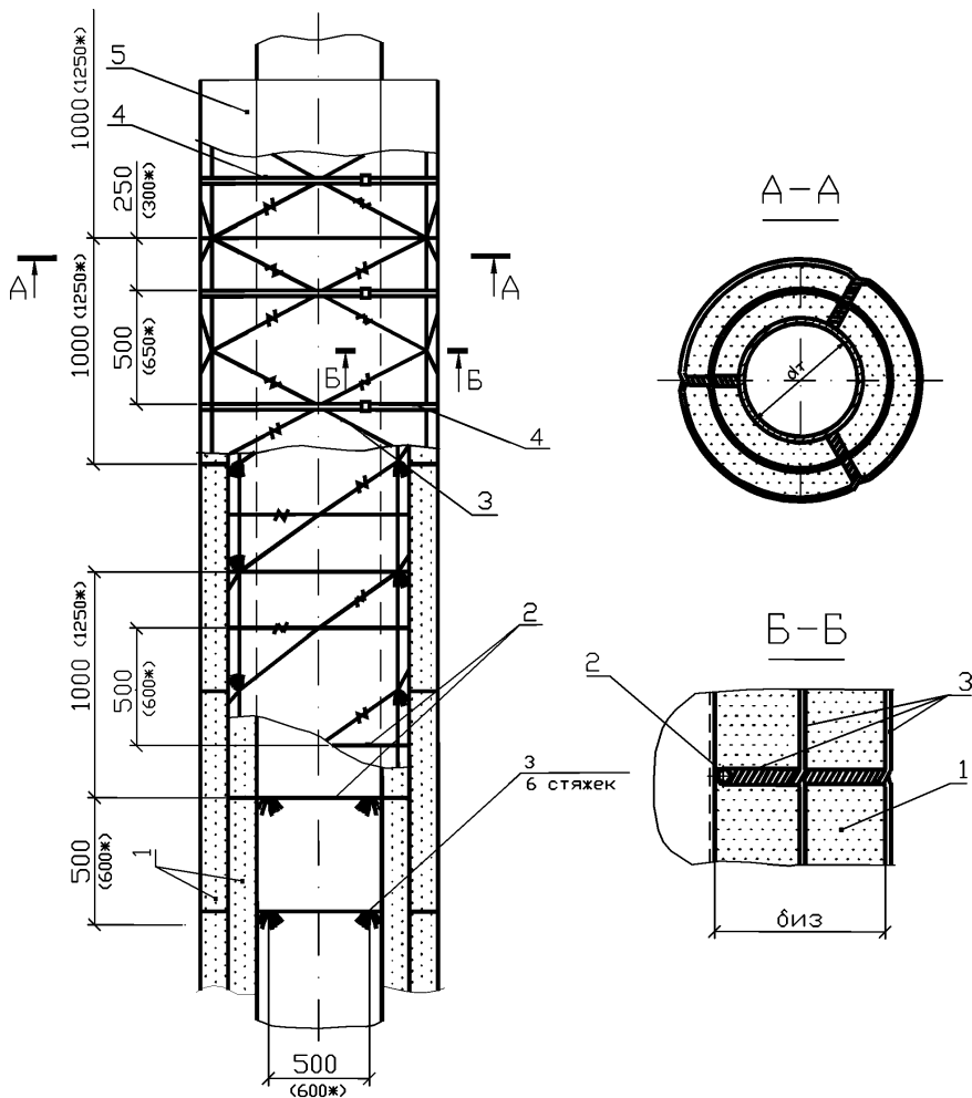
Рис. 8.6 Изоляция трубопроводов наружным диаметром 530 мм и более теплоизоляционными изделиями URSA® в два слоя с креплением
