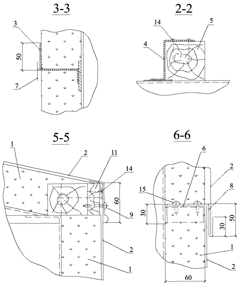
Рис. 4.23 Разрезы 2-2, 3-3, 5-5 и 6-6 к рис.4.21
