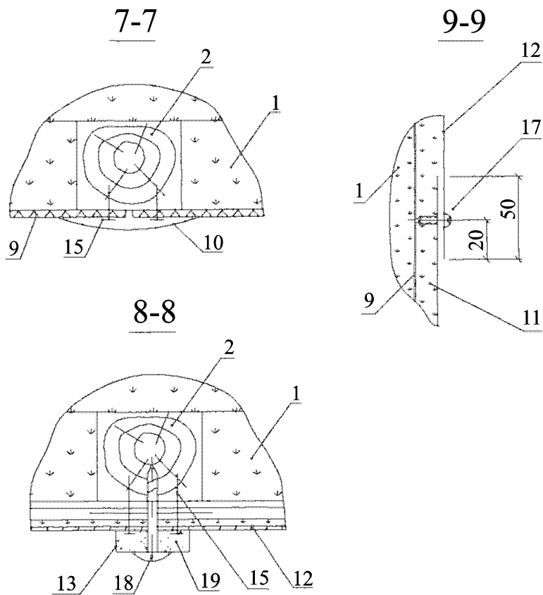
Рис. 4.29 Разрезы 7-7 и 9-9 к рис.4.25
