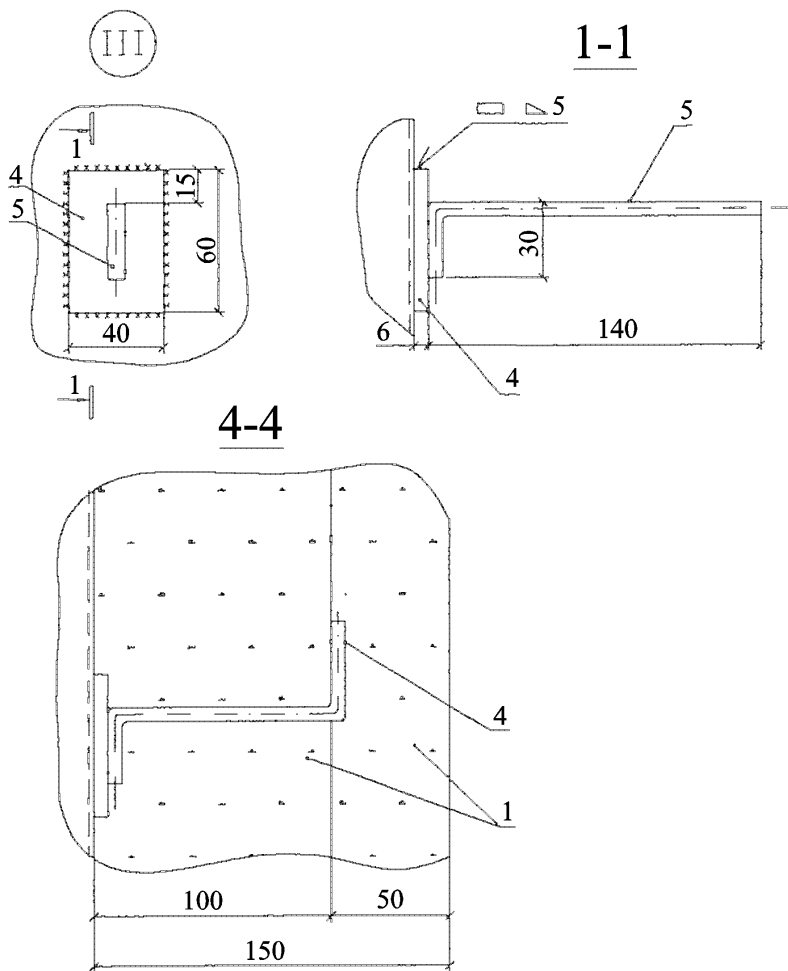
Рис. 4.26 Узел III и разрез 4-4 к рис.4.25
