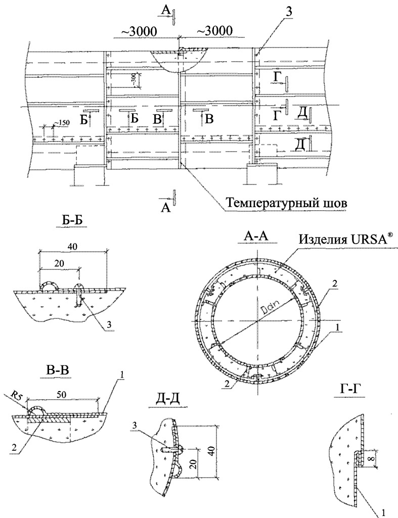
Рис. 4.12 Конструкция защитного покрытия тепловой изоляции горизонтального аппарата
