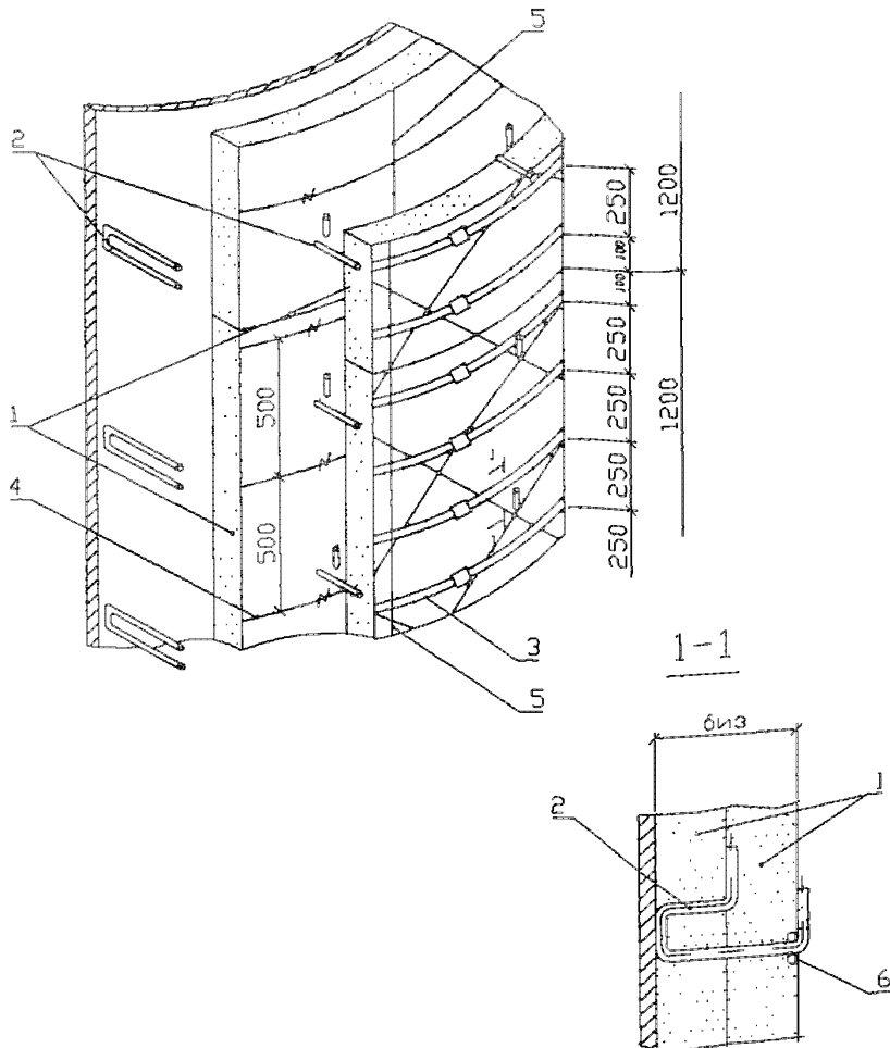
Рис. 4.8 Конструкция тепловой изоляции на основе матов URSA® М-25 в два слоя с креплением штырями, бандажами и стяжками
