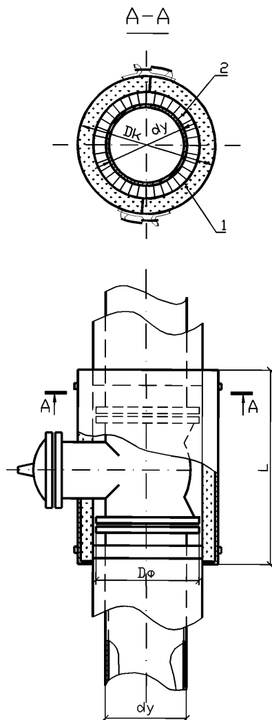
Рис. 8.12 Изоляция арматуры съемной конструкцией с теплоизоляционным слоем из матов теплоизоляционных URSA® (полуфутляры)
