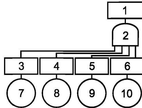
Рисунок 3 — Представление параллельной системы в виде ДН
