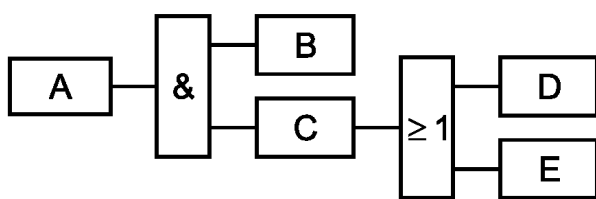
Рисунок 5 — Представление вентиляей и событий в виде прямоугольников
