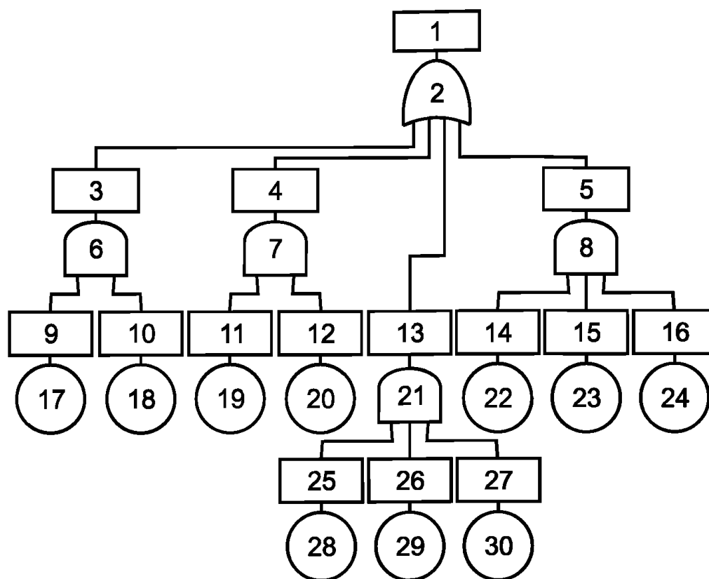
1 — вероятность отказа мостовой схемы; 2 — мостовая схема; 3 — прерывание сигнала блоками A и B; 4 — прерывание сигнала блоками C и D; 5 — прерывание сигнала блоками B, E и C; 6 — блоки A и B; 7 — блоки C и D; 8 — блоки B, E и C; 9 — событие отказа блока A; 10 — событие отказа блока B; 11 — событие отказа блока C; 12 — событие отказа блока D; 13 — прерывание сигнала блоками A, E и D; 14 — событие отказа блока B; 15 — событие отказа блока E; 16 — событие отказа блока C; 17 — блок A; 18 — блок B; 19 — блок C; 20 — Блок D; 21 — блоки A, E и D; 22 — блок B; 23 — блок E; 24 — блок C; 25 — событие отказа блока A; 26 — событие отказа блока E; 27 — событие отказа блока D; 28 — блок A; 29 — блок E; 30 — блок D
