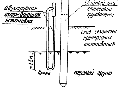
Свайный или стальной фундамент с двухтрубной охлаждающей установкой
