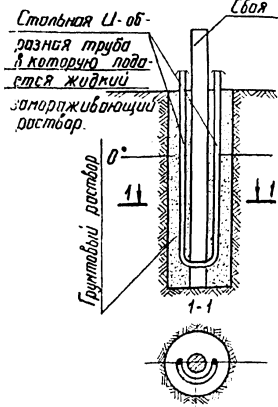
Свая с трубой для машинного охлаждения грунтового раствора и основания
