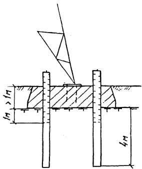
Фундамент с использованием металлических свай в качестве охлаждающих установок
