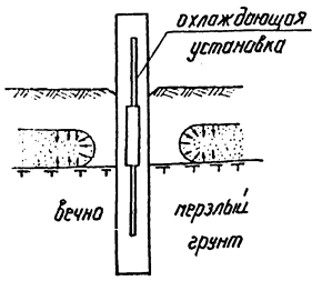
Фундамент с размещенной внутри охлаждающей установкой
