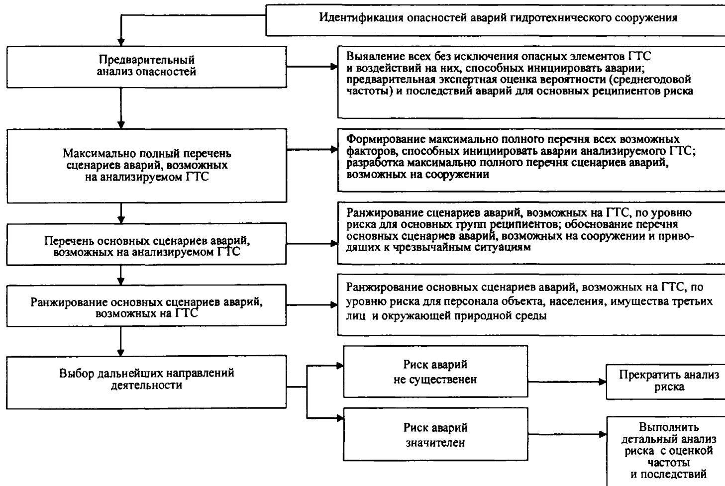
Рис. 3. Основные шаги процедуры идентификации опасностей
