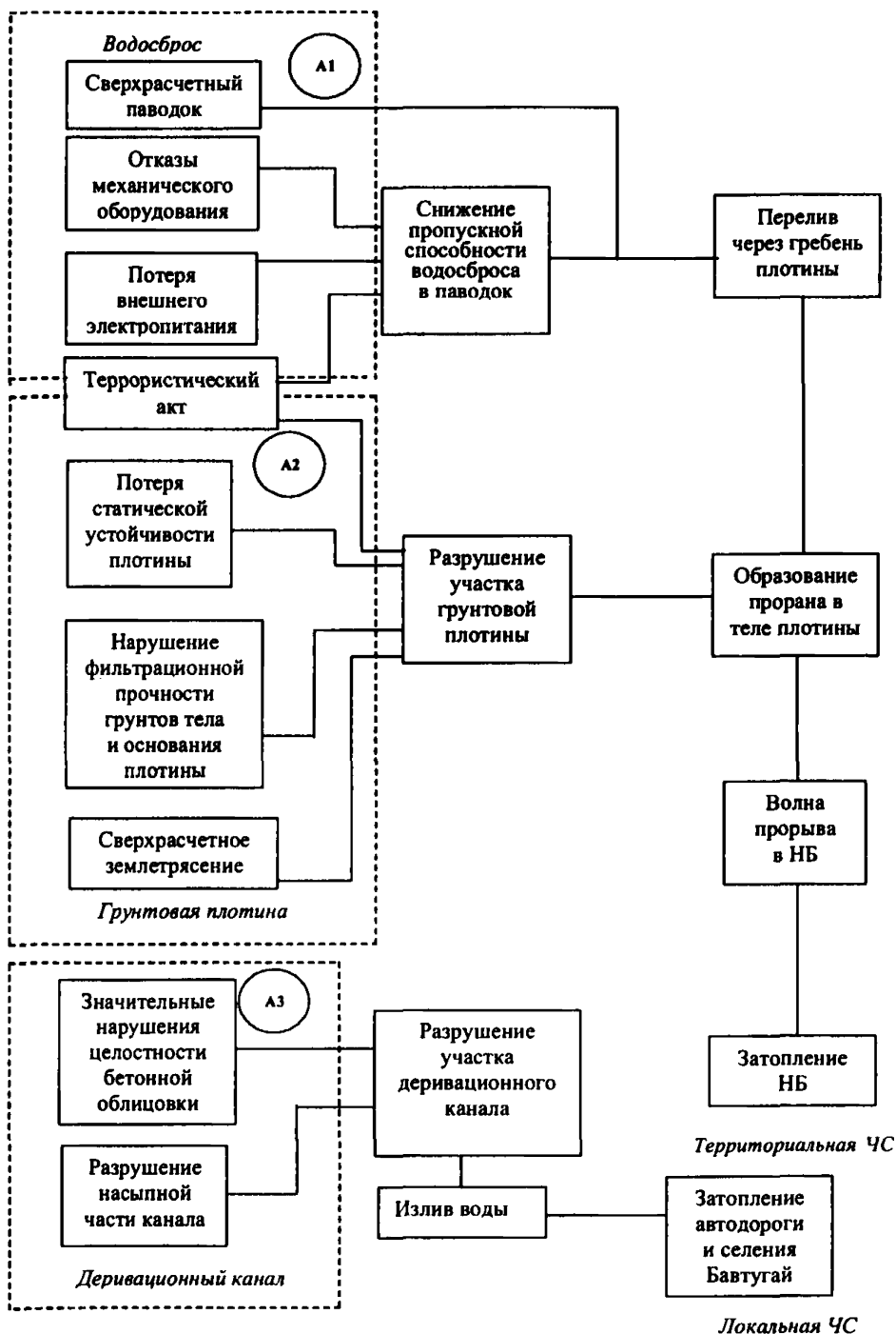
Рис. П2.1. Блок-схема анализа основных вероятных сценариев возникновения и развития аварий на ГЭС Чирчуртских ГЭС
