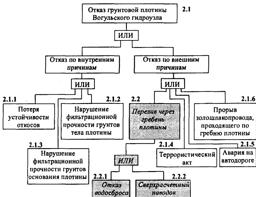
Рис. П2.13. «Дерево отказов» для сценариев 2.1 и 2.2 аварии ГЭС
