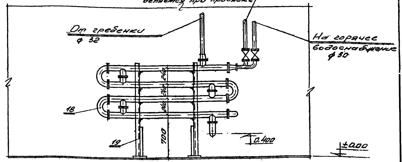
РАЗРЕЗ II-II
