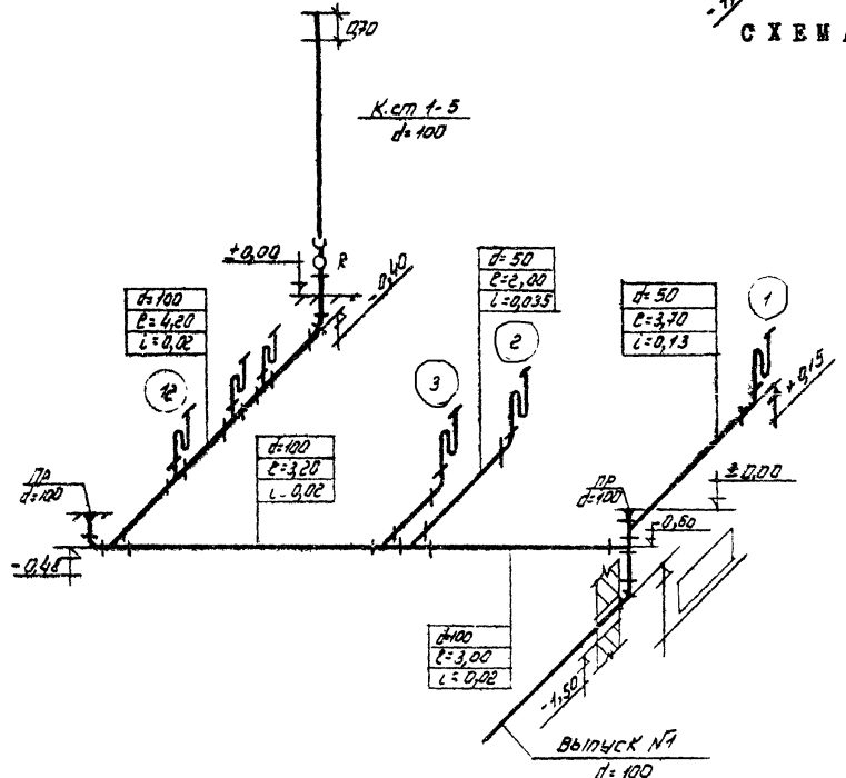
СХЕМА СЕТИ ПРОИЗВОДСТВЕННОЙ КАНАЛИЗАЦИИ
