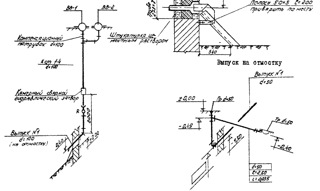
СХЕМА СЕТИ ВНУТРЕННИХ ВОДОСТОКОВ
